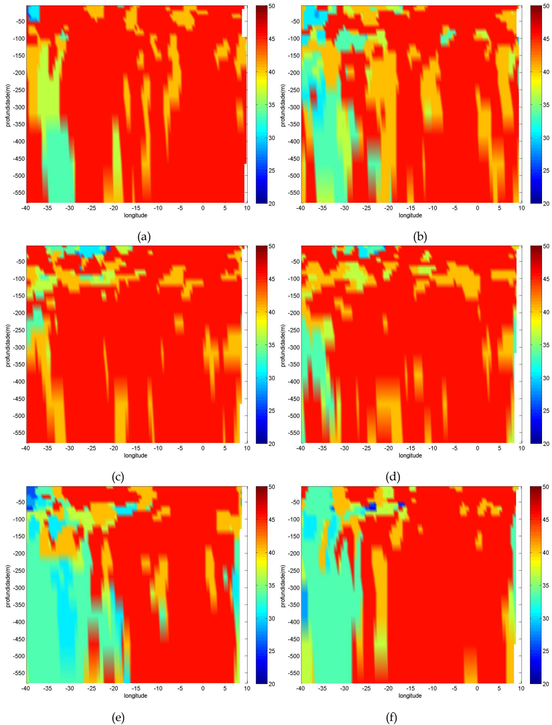
Figura 4.38: Períodos dominante (em dias) no sinal da componente zonal de corrente, filtrado entre 5 e 25° de longitude e 20 e 50 dias, nas seções verticais ao longo da latitude de 2,25°N (a), 1,25°N (b), 0,25°N (c), 0,25°S (d), 1,25°S (e) e 2,25°S (f).
