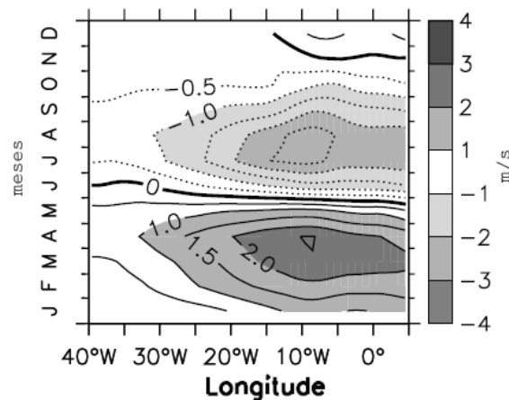
Figura 2.10: Ciclo sazonal de TSM. Adaptado de: Ding et al (2009).
