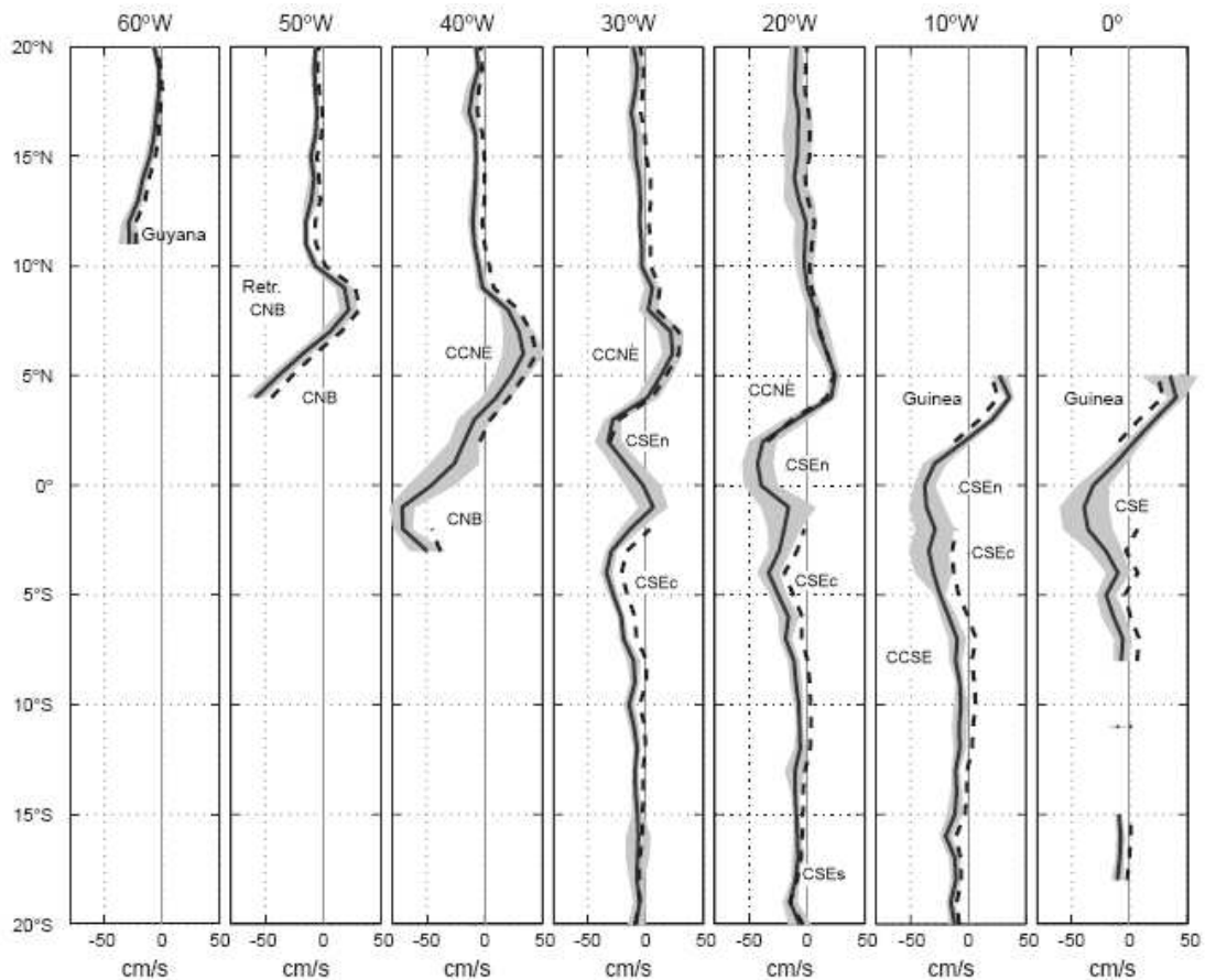
Figura 2.8: Curva sólida: média anual de velocidade zonal de derivadores (média zonal a cada 5°). Sombreado: erro padrão. Adaptado de: Lumpkin e Garzoli (2005).
