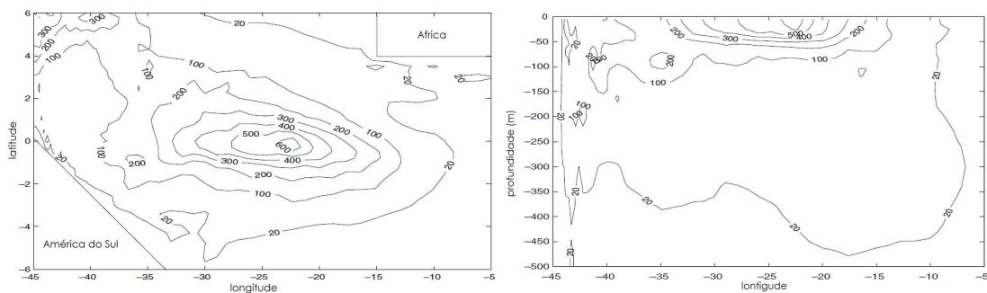
Figura 2.14: Distribuição espacial da energia cinética da perturbação (média do período), extraída do modelo e filtrada no período de 20 - 50 dias (contornos em \text{cm}^2/\text{s}^2 ). Adaptado de: Jochum et al (2004b).
