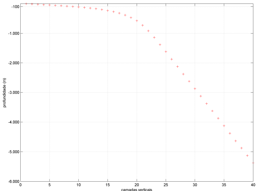
Figura 3.2: Discretização vertical do SODA 2.1.6.
