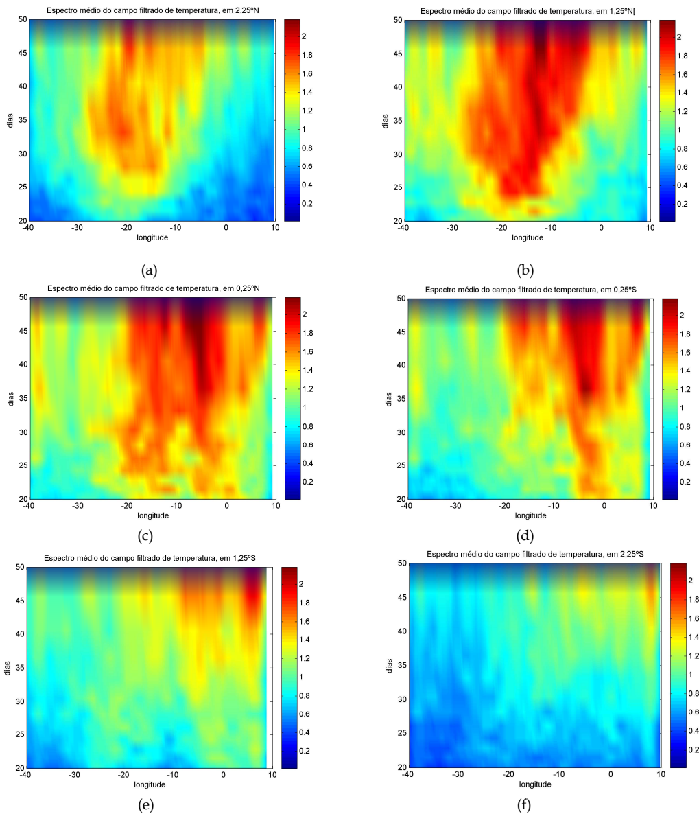
Figura 4.33: Espectro anual médio do campo de temperatura, filtrado entre 5 e 25^{\circ} de longitude e 20 e 50 dias, em 2,25^{\circ}\text{N} (a), 1,25^{\circ}\text{N} (b), 0,25^{\circ}\text{N} (c), 0,25^{\circ}\text{S} (d) 1,25^{\circ}\text{S} (e) e 2,25^{\circ}\text{S} (f).
