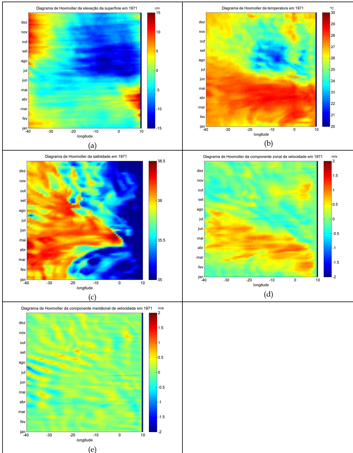
Figura 4.10: Diagramas de Hovmöller dos resultados do SODA na primeira camada (cerca de 5 metros de profundidade), ao longo da latitude de 0,25°N, durante o ano de 1971. (a) elevação da superfície livre (cm), (b) temperatura (°C), (c) salinidade (d) componente zonal (m/s) e (e) meridional da velocidade (m/s).
