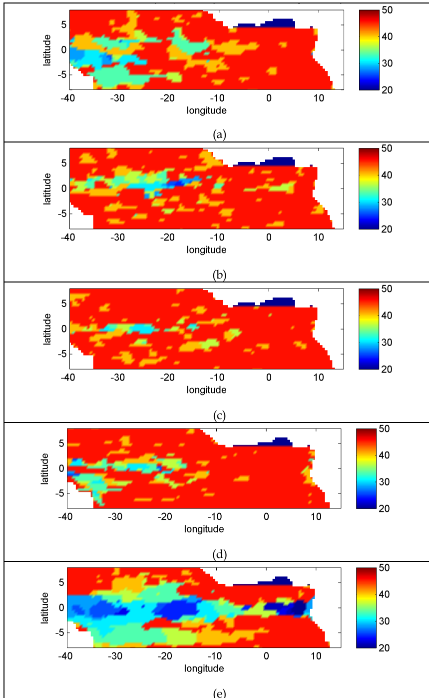
Figura 4.29: Períodos dominantes (em dias) nos sinais de elevação da superfície livre (a), temperatura (b), salinidade (c) e componente zonal (d) e meridional (e) de corrente, filtrados entre 5 e 25° de longitude e 20 e 50 dias.
