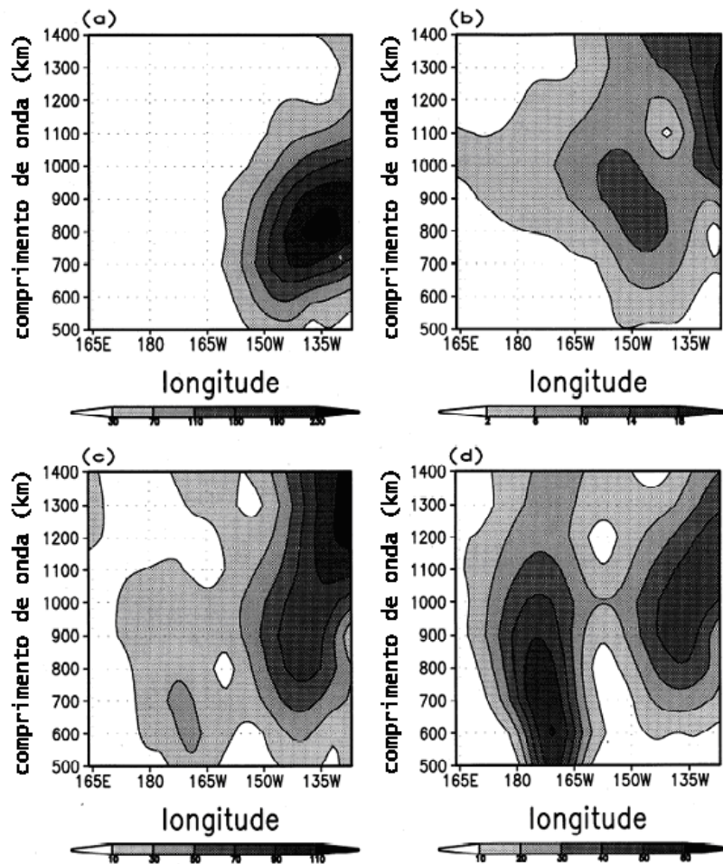
Figura 2.26: Módulo do coeficiente da transformada de ondeleta da velocidade meridional, na latitude 2°N em 5 metros (a) e 713 metros (b) de profundidade, e na latitude 2°S em 5 metros (c) e 713 metros (d) de profundidade. O intervalo do contorno está em cm/s de acordo com a escala de cores. Os maiores valores representados na escala de cor indicam alta correlação entre os dados e a ondeleta. Adaptado de: Masina e Philander (1999).
