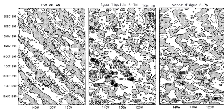
Figura 2.32: Seções de longitude x tempo de anomalia de TSM em 4°N, água líquida e vapor d'água. Adaptado de: Hashizume et al (2001).
