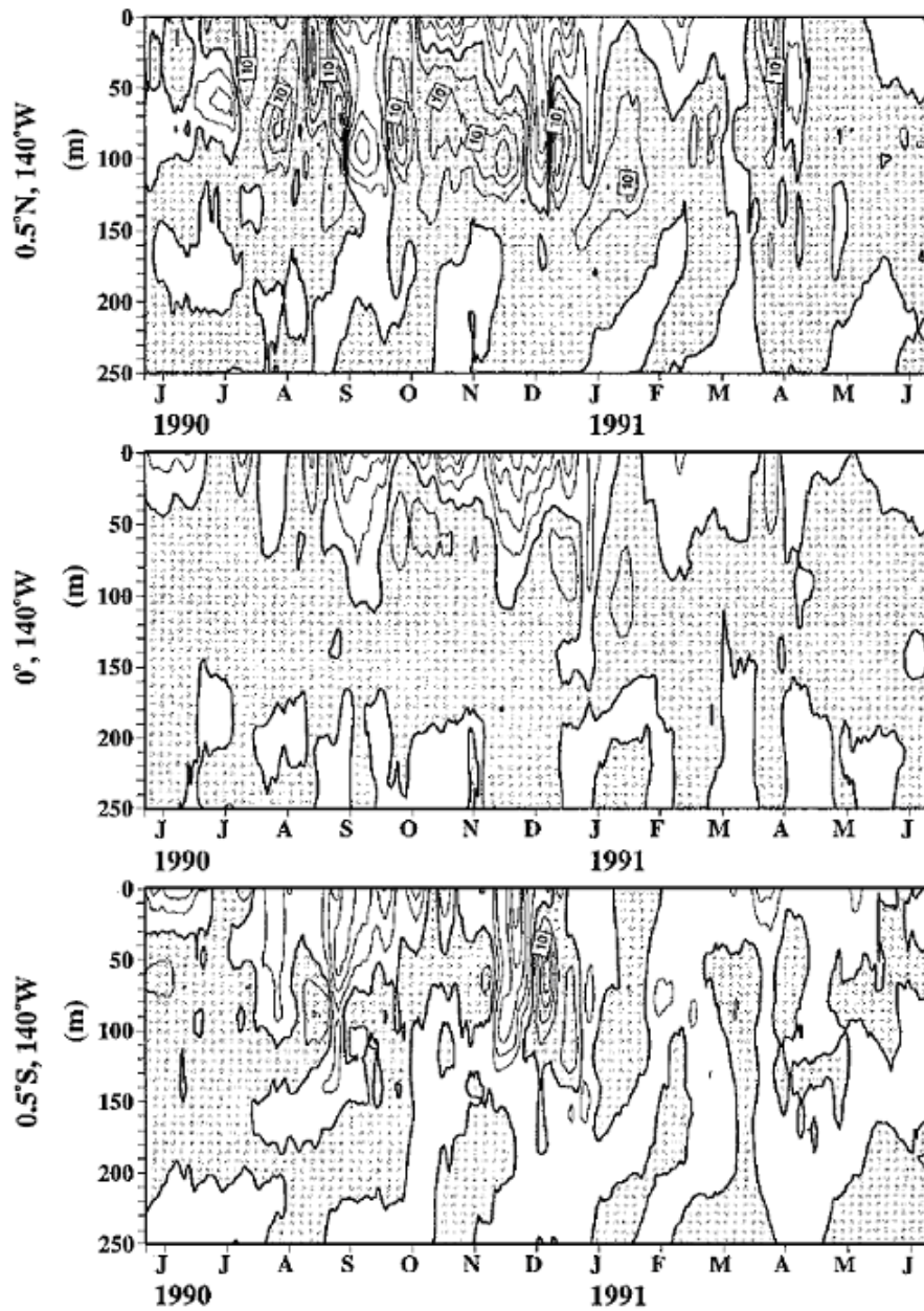
Figura 2.22: Soma dos dois principais termos de trabalho de deformação -(\overline{u'vU_y} + \overline{v'vV_y}) em função do tempo e profundidade. Valores positivos estão sombreados e o intervalo dos contornos é 5 \times 10^{-4} \text{ cm}^2\text{s}^{-3} . Fonte: Qiao e Weisberg (1998).
