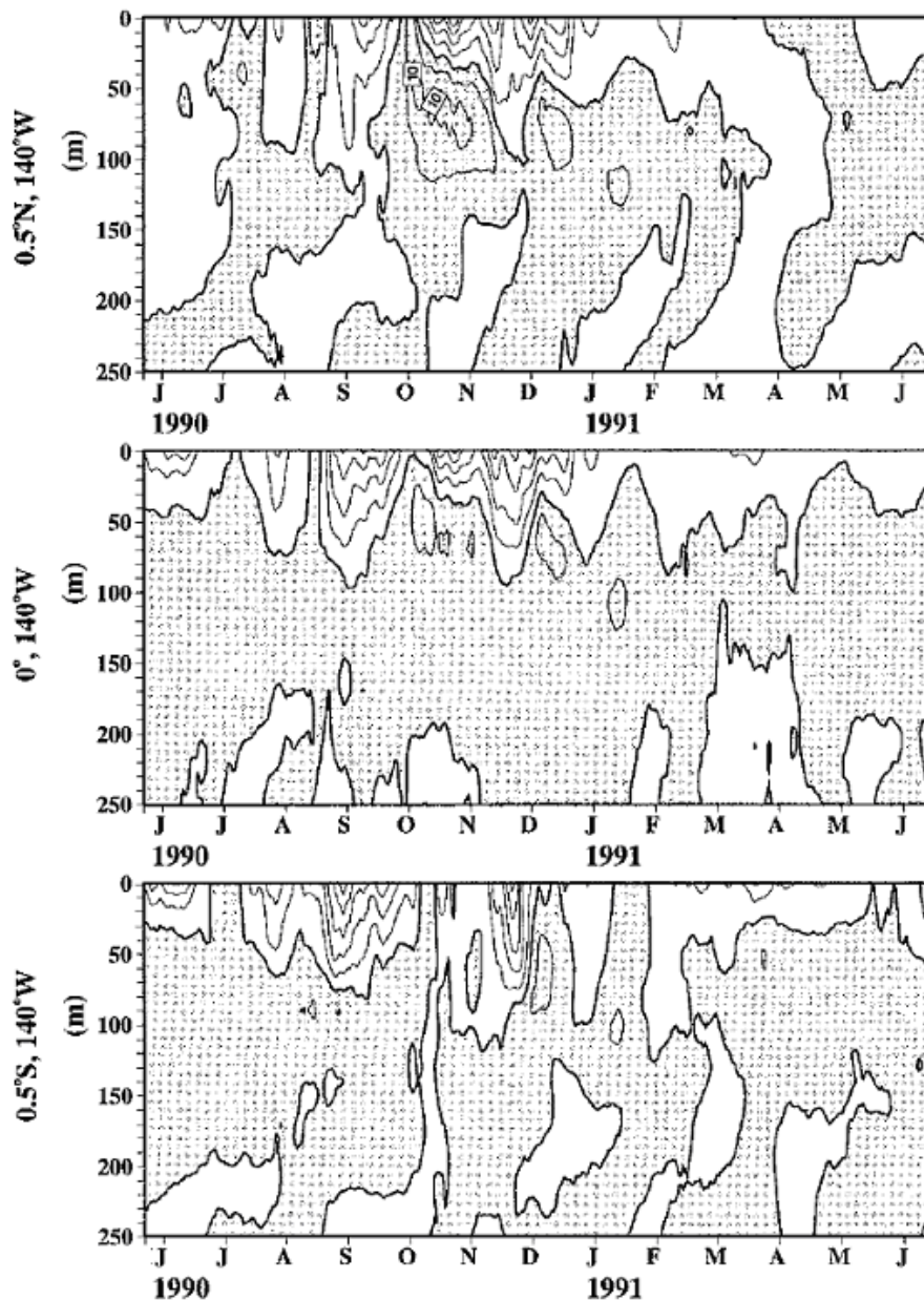
Figura 2.23: Termo de trabalho de deformação -\overline{v'v_y} , em função do tempo e profundidade. Valores positivos estão sombreados e o intervalo dos contornos é 5 \times 10^{-4} \text{ cm}^2\text{s}^{-3} . Fonte: Qiao e Weisberg (1998).
