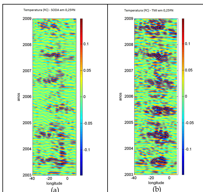
Figura 4.16: Temperatura na primeira camada (cerca de 5 metros de profundidade) do SODA (a) e TSM do TMI/AMSRE, ambos filtrados para o período entre 20 a 50 dias, e 5^{\circ} e 25^{\circ} de longitude, ao longo da latitude de 0,25^{\circ}\text{N} , entre 2003 e 2008.
