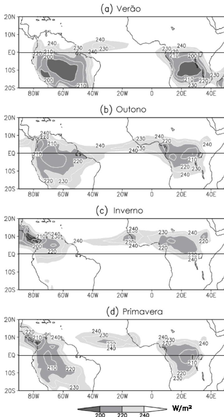
Figura 2.3: Média climatológica da radiação de onda longa emitida para o espaço no período de 1979 - 1993, sobre o Atlântico tropical ilustrando o posicionamento da ZCIT ao longo do ano. Adaptado de: Wang e Fu (2007).
