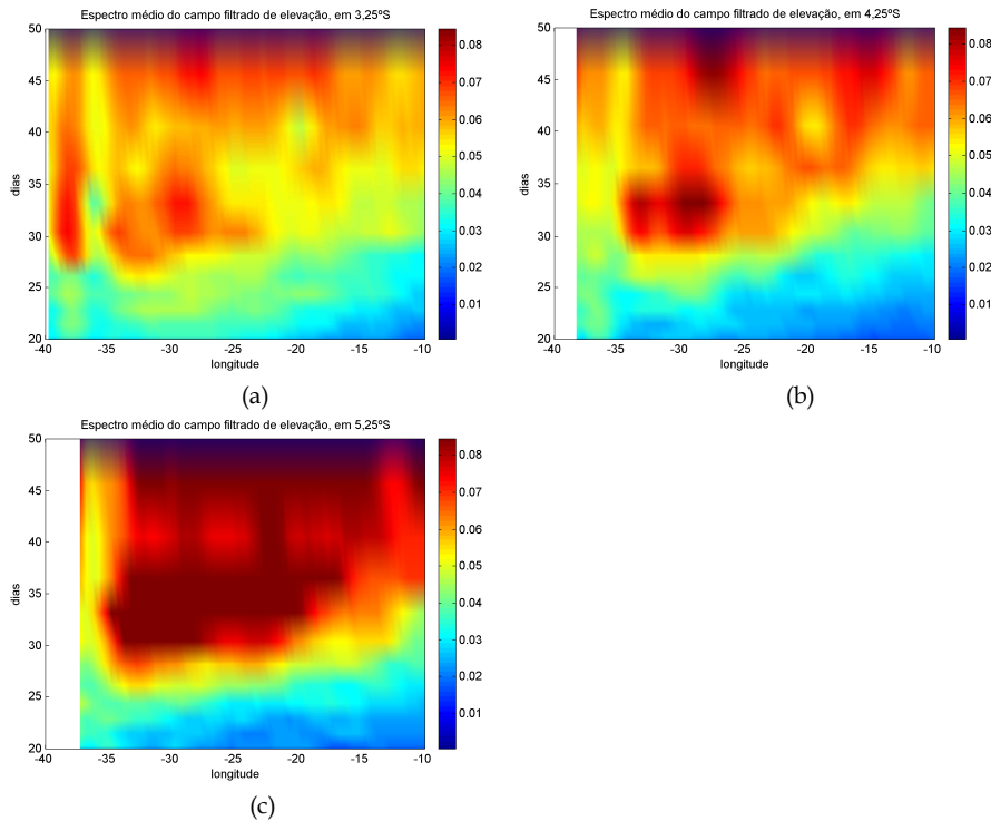
Figura 4.32: Espectro anual médio do campo de elevação da superfície livre, filtrado entre 5 e 25° de longitude e 20 e 50 dias, em 3,25°S (a), 4,25°S (b) e 5,25°S (c).
