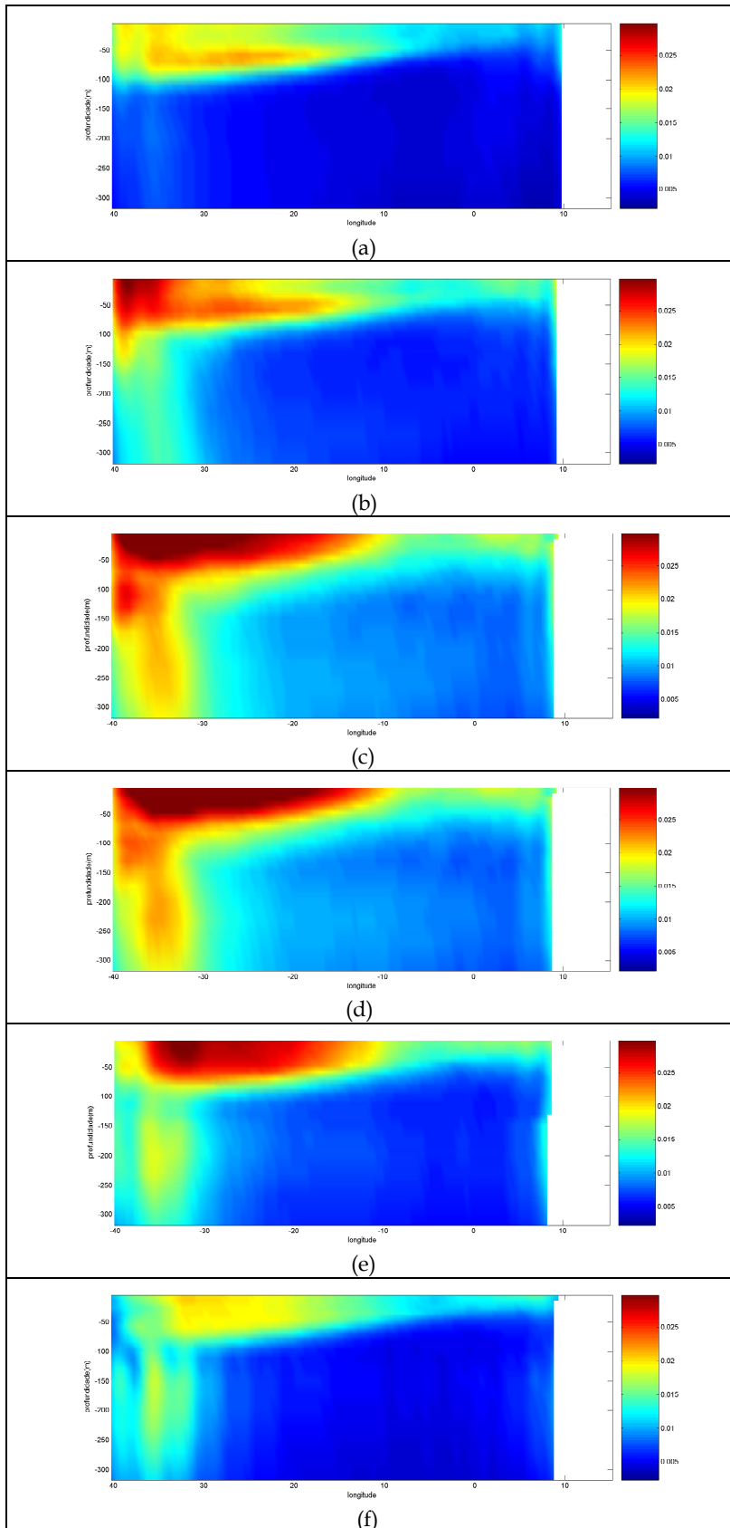
Figura 4.28: Desvio padrão do sinal das OITs no campo da componente meridional de corrente (m/s) do SODA, filtrado para o período entre 20 a 50 dias, e 5° e 25° de longitude, entre a superfície e 330 metros, ao longo das latitudes de 2,25°N (a), 1,25°N (b), 0,25°N (c), 0,25°S (d), 1,25°S (e) e 2,25°S (f).
