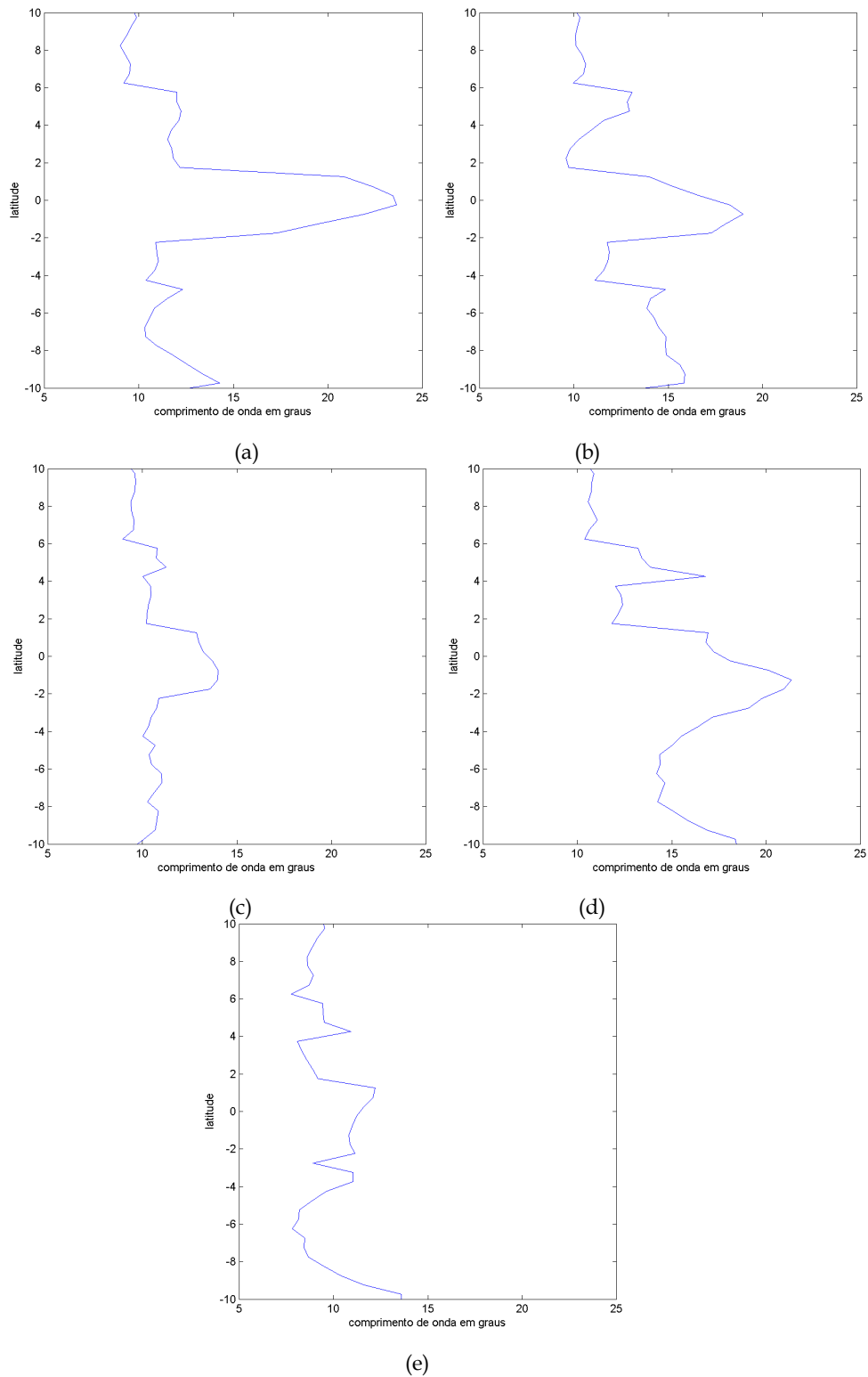
Figura 4.41: Comprimento de onda dominante (em graus) na região entre 40,25^{\circ}\text{W} e 10,25^{\circ}\text{W} , na camada superficial, nos sinais de elevação da superfície livre (a), temperatura (b), salinidade (c) e componente zonal (d) e meridional (e) de corrente, filtrados entre 5 e 25^{\circ} de longitude e 20 e 50 dias.
