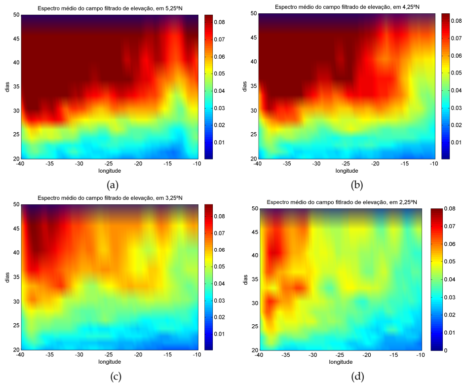
Figura 4.30: Espectro anual médio do campo de elevação da superfície livre, filtrado entre 5 e 25° de longitude e 20 e 50 dias, em 5,25°N (a), 4,25°N (b), 3,25°N (c), 2,25°N (d).
