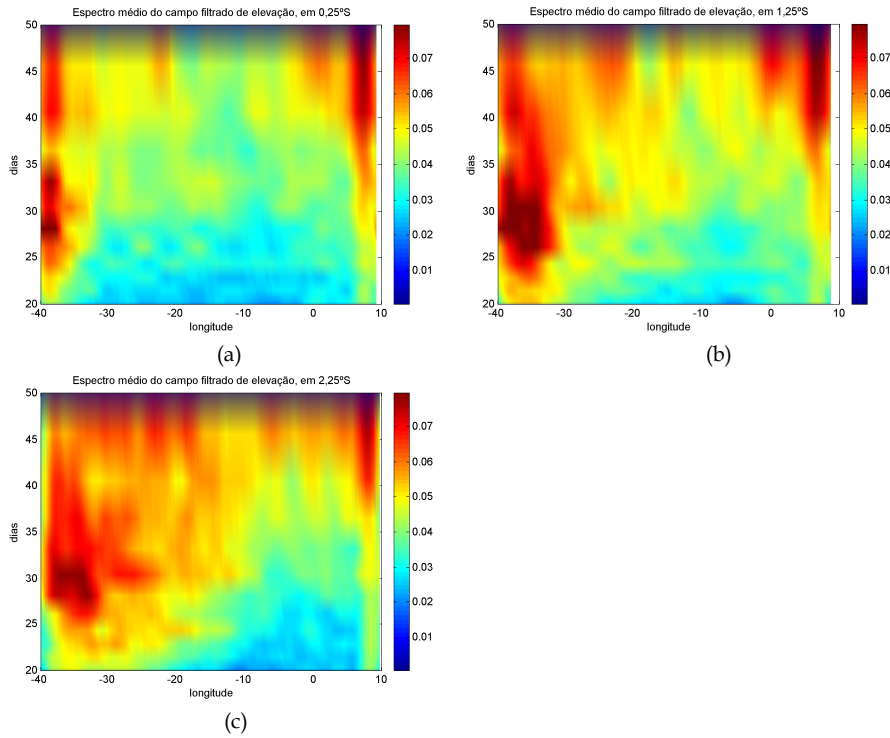
Figura 4.31: Espectro anual médio do campo de elevação da superfície livre, filtrado entre 5 e 25° de longitude e 20 e 50 dias, em 0,25°S (a), 1,25°S (b) e 2,25°S (c).
