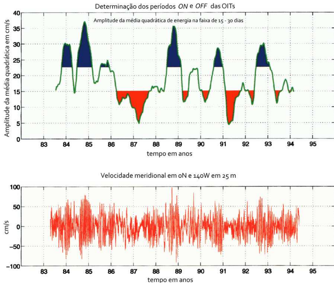
Figura 2.20: Índice de ocorrência das OITs no Pacífico em 0°N e 140°W. A linha verde é a amplitude da média quadrática da energia na faixa de 15-30 dias. As colorações azul e vermelha correspondem aos períodos on e off , respectivamente. Adaptado de: Baturin e Niiler (1997).
