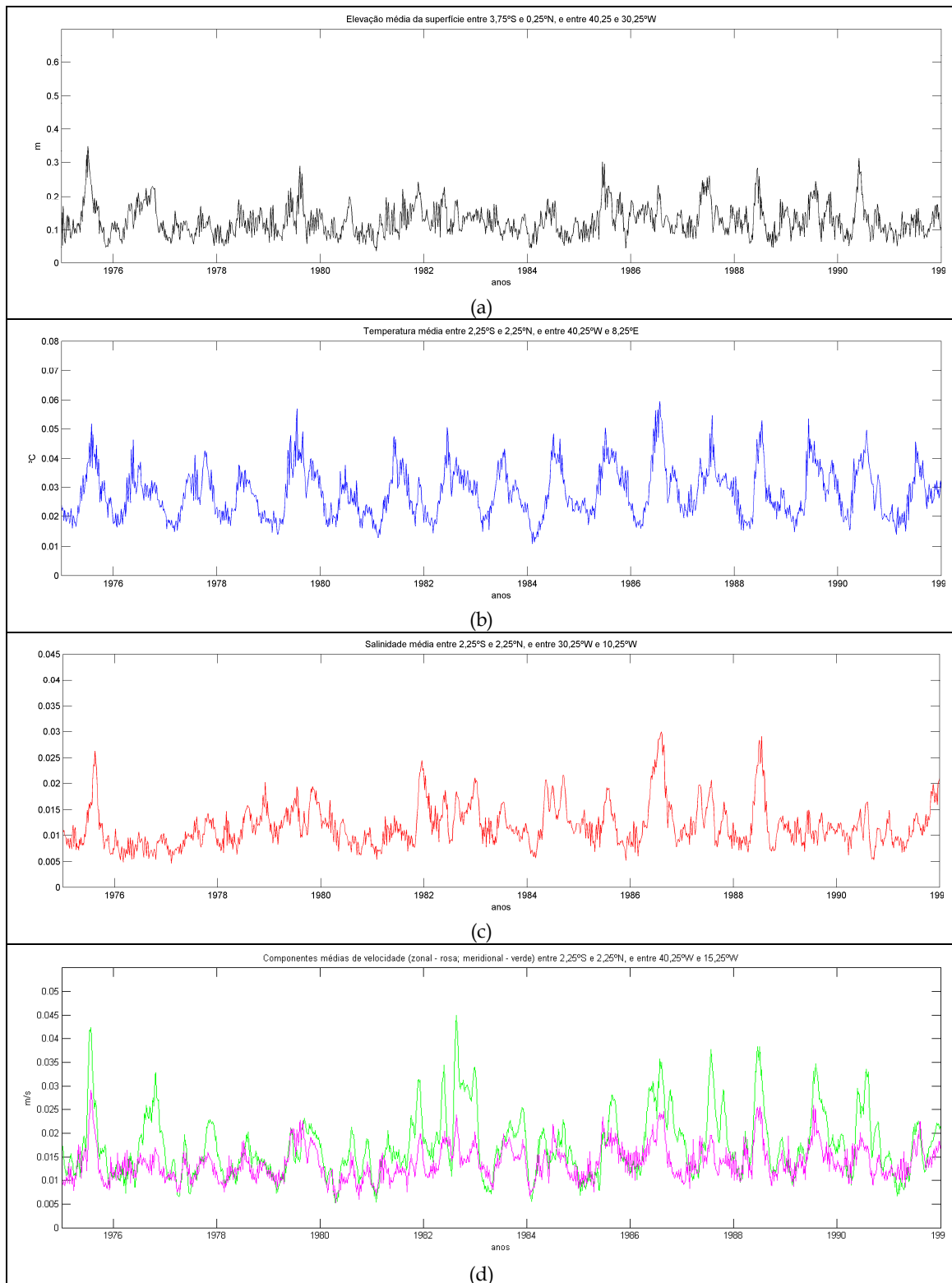
Figura 4.52: Valores médios das variáveis nas regiões de maior desvio padrão dos campos filtrados, entre os anos de 1975 e 1991. Média da elevação da superfície livre na região entre as os limites de 3,75°S a 0,25°N e 40,25°W a 30,25°W (a), média da temperatura entre os limites de 2,25°S a 2,25°N e 40,25°W a 8,25°E (b), média da salinidade entre os limites de 2,25°S a 2,25°N e 30,25°W a 10,25°W (c), e média das componentes zonal (rosa) e meridional (verde) da velocidade entre os limites de 2,25°S a 2,25°N e 40,25°W a 15,25°W.
