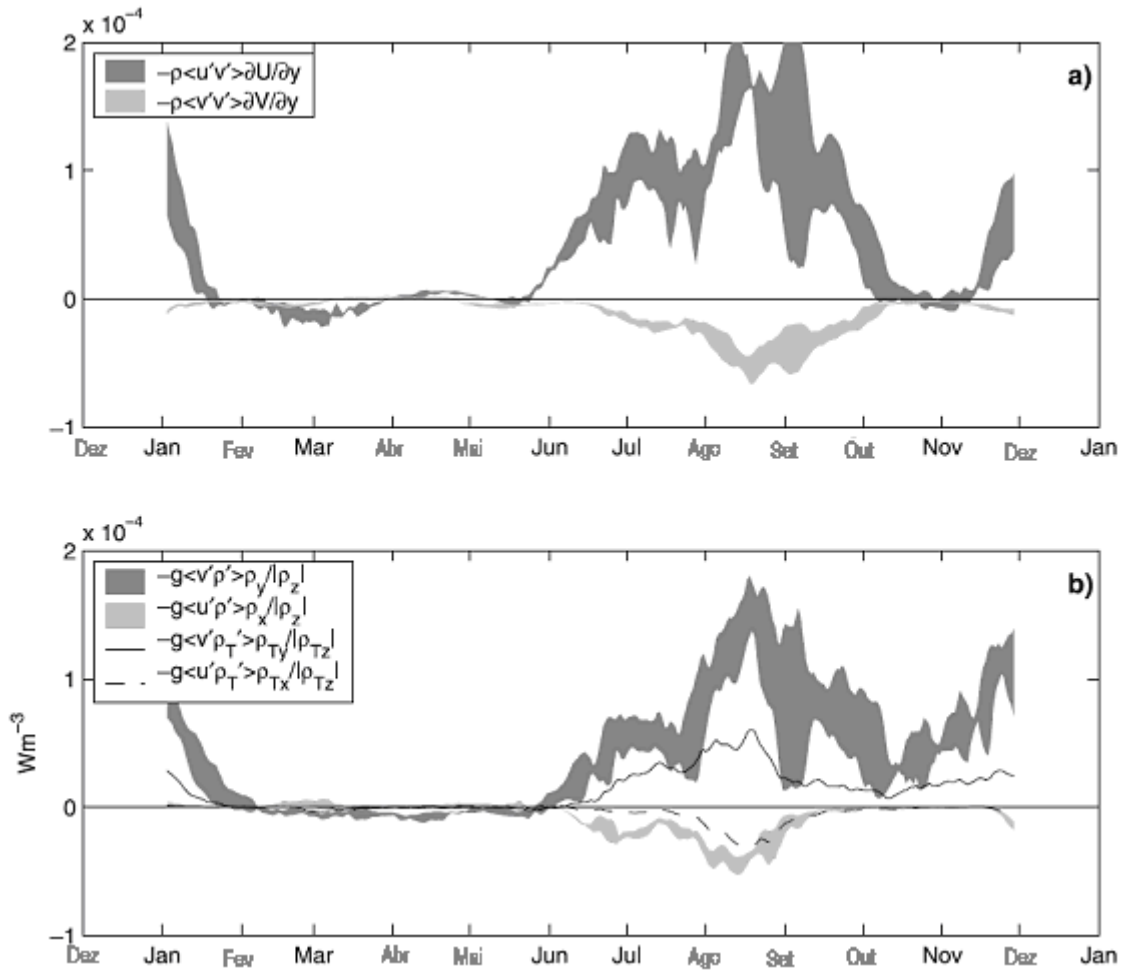
Figura 2.16: (a) Conversão barotrópica de energia nos primeiros 40 metros de profundidade. As sombras mostram o espalhamento das estimativas baseadas nas médias móveis de 20, 30 e 40 dias. (b) O mesmo que em (a), mas para conversão baroclínica. As linhas em (b) demonstram as conversões de energia somente considerando a temperatura, sem a salinidade. Adaptado de: Grodsky et al (2005).
