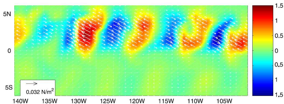
Figura 2.34: Atrito do vento (vetores) e TSM (colorido, em °C) filtrados. Fonte: Pezzi et al (2004).
