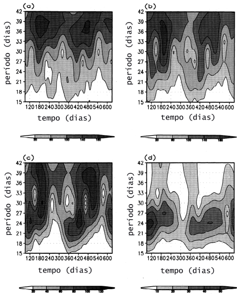
Figura 2.25: Módulo do coeficiente da transformada de ondeleta da velocidade meridional, em 110°W, na latitude 2°N em 5 metros (a), 75 metros (b), 113 metros (c) e 713 metros (d) de profundidade. O intervalo do contorno está em cm/s de acordo com a escala de cores. Os maiores valores representam na escala de cor indicam alta correlação entre os dados e a ondeleta. Adaptado de: Masina e Philander (1999).
