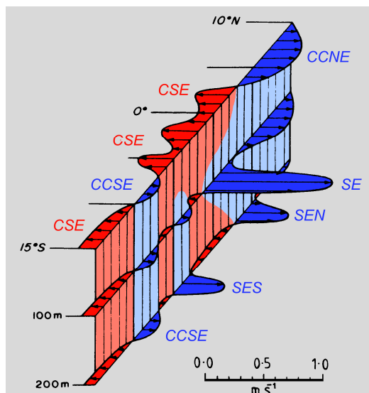
Figura 2.9: Esquema da estrutura do sistema de correntes oceânicas equatoriais do Atlântico. Adaptado de: Tomczak e Godfrey (2005).
