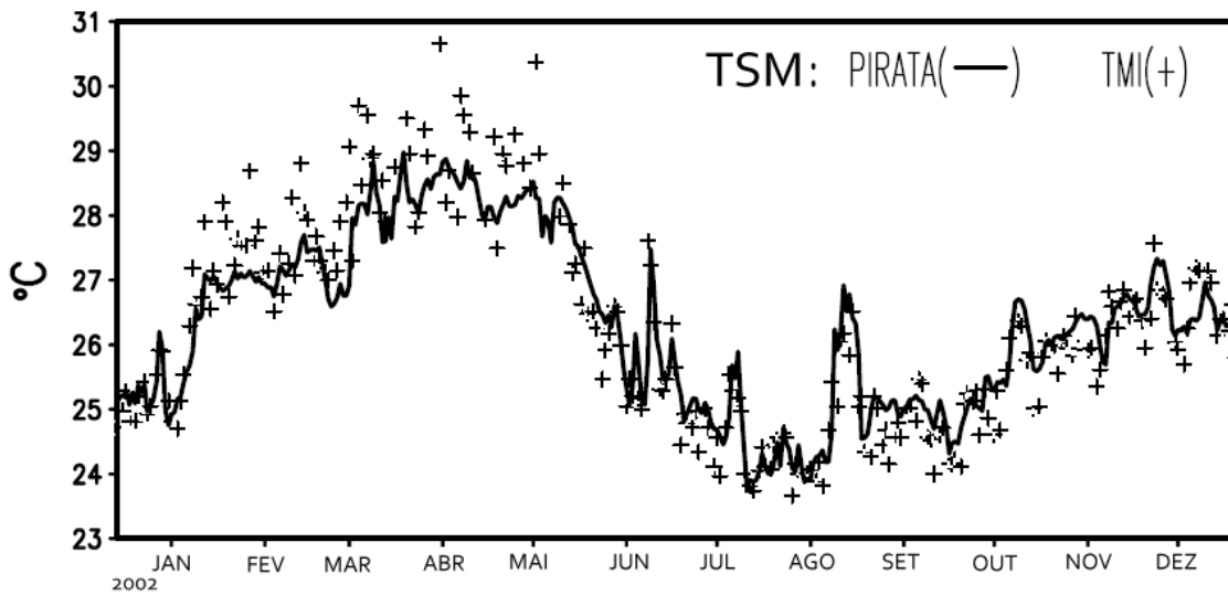
Figura 2.15: Comparação da série de TSM média de 3 dias medida pela bóia do PIRATA e pelo sensor do TMI. Adaptado de: Grodsky et al (2005).
