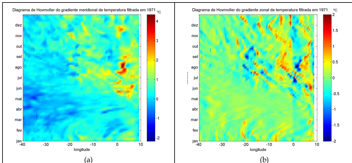
Figura 4.11: Diagramas de Hovmöller dos gradientes meridional (a) e zonal (b) da temperatura (em °C) gerada pelo SODA na primeira camada (cerca de 5 metros de profundidade), ao longo da latitude de 0,25°N, durante o ano de 1971.
