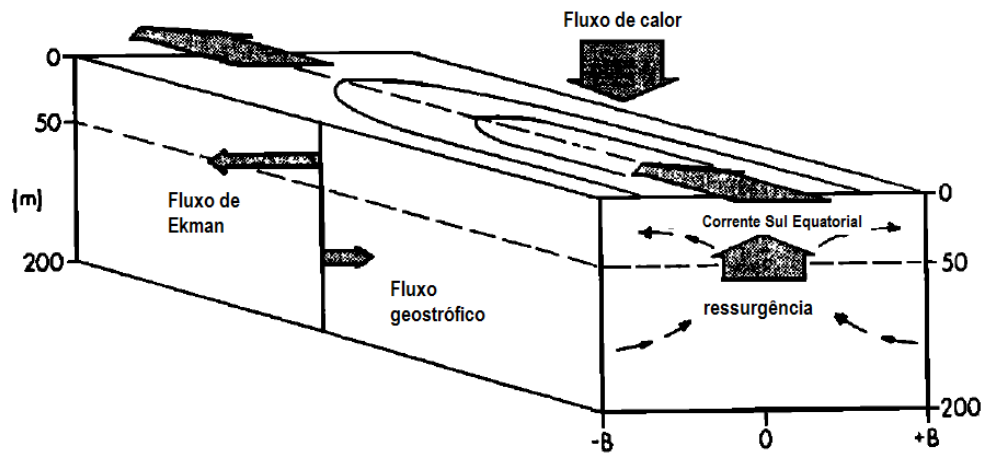
Figura 2.5: Representação esquemática dos principais componentes do balanço de massa e calor na região equatorial. Adaptado de: Wyrtki (1981), apud Lee e Csanady (1999).
