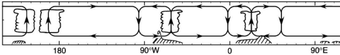
Figura 2.1: Célula equatorial zonal de circulação atmosférica. Fonte: Holton (2004).
