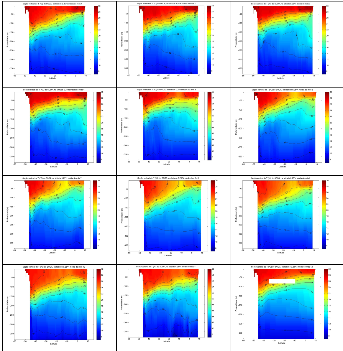
Figura 4.2: Médias mensais de temperatura (em graus Celsius) gerada pelo SODA na seção zonal vertical ao longo da latitude de 0,25^{\circ}\text{N} .
