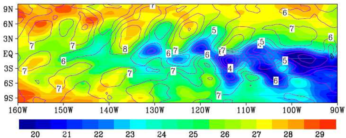
Figura 2.30: Temperatura da superfície do mar (colorido, em °C) estimada pelo TMI e velocidade do vento em superfície (contorno, em m/s) estimado pelo SeaWinds em 11 de setembro de 1999. Fonte: Liu et al (2000).
