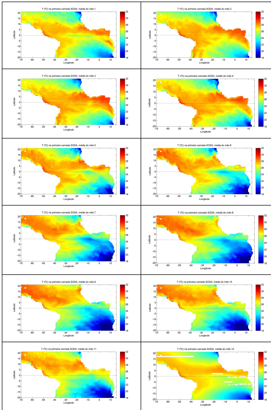
Figura 4.1.: Médias mensais de temperatura (em graus Celsius) na primeira camada do SODA.
