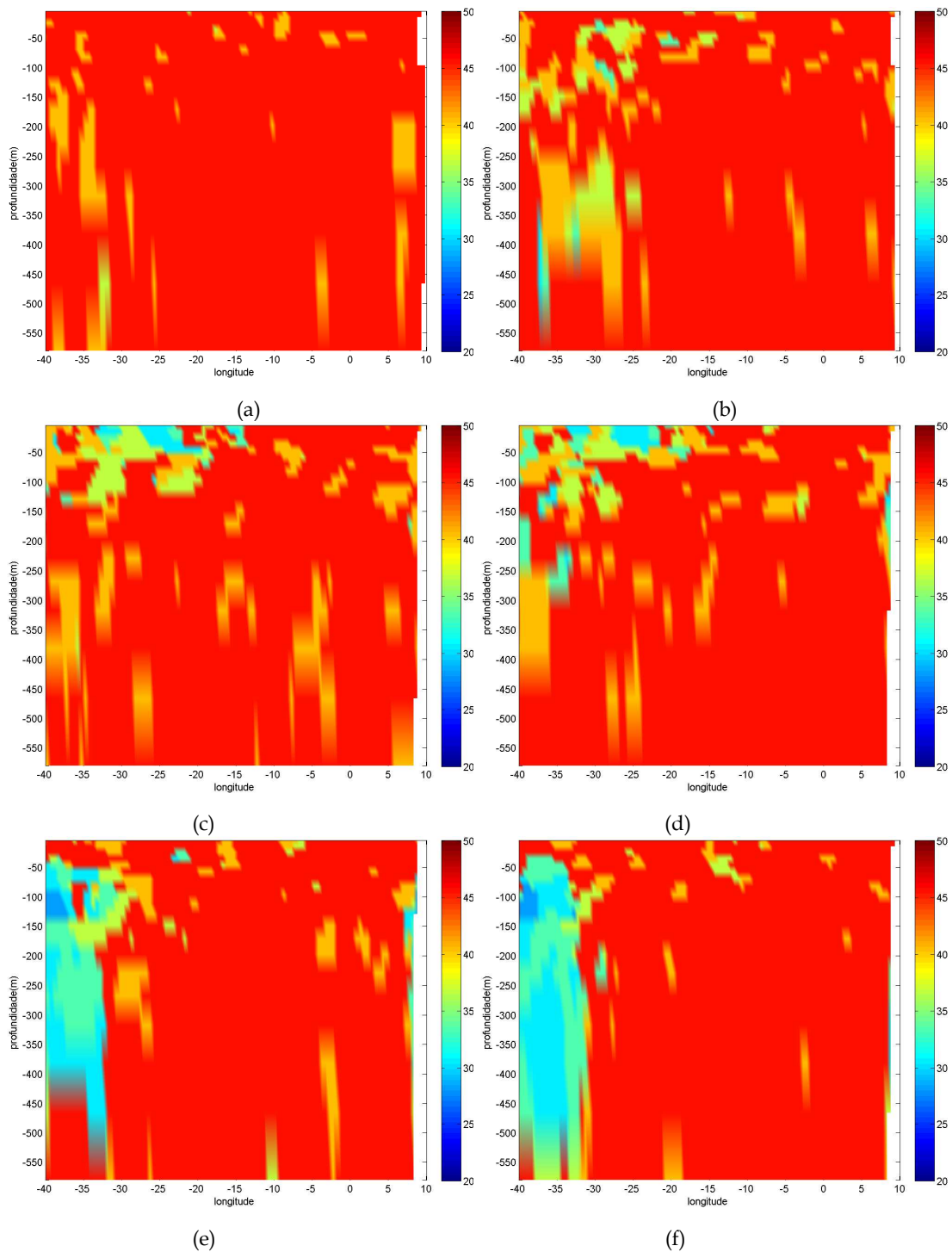
Figura 4.37: Períodos dominantes (em dias) no sinal de salinidade filtrado entre 5 e 25° de longitude e 20 e 50 dias, nas seções verticais ao longo da latitude de 2,25°N (a), 1,25°N (b), 0,25°N (c), 0,25°S (d), 1,25°S (e) e 2,25°S (f).
