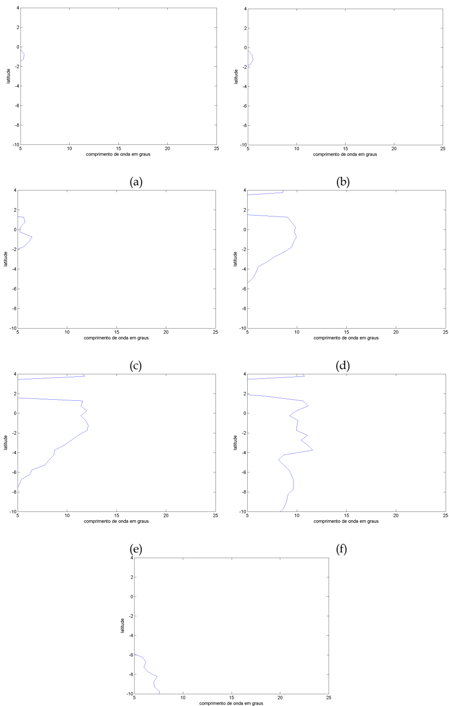
(g) Figura 4.47: Comprimento de onda dominante (em graus) na região entre 15,25°W e 15,25°E, no sinal de temperatura, filtrado entre 5 e 25° de longitude e 20 e 50 dias, a 15 (a), 35 (b), 46 (c), 83 (d), 96 (e), 148 (f) e 229 (g) metros de profundidade.
