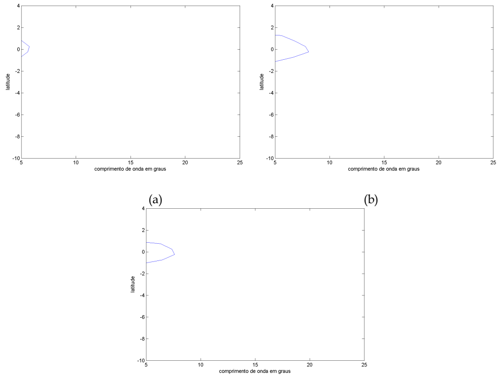
Figura 4.50: Comprimento de onda dominante (em graus) na região entre 15,25°W e 15,25°E, no sinal da componente meridional de corrente, filtrado entre 5 e 25° de longitude e 20 e 50 dias, a 46 (a), 83 (b) e 96 (c) metros de profundidade.
