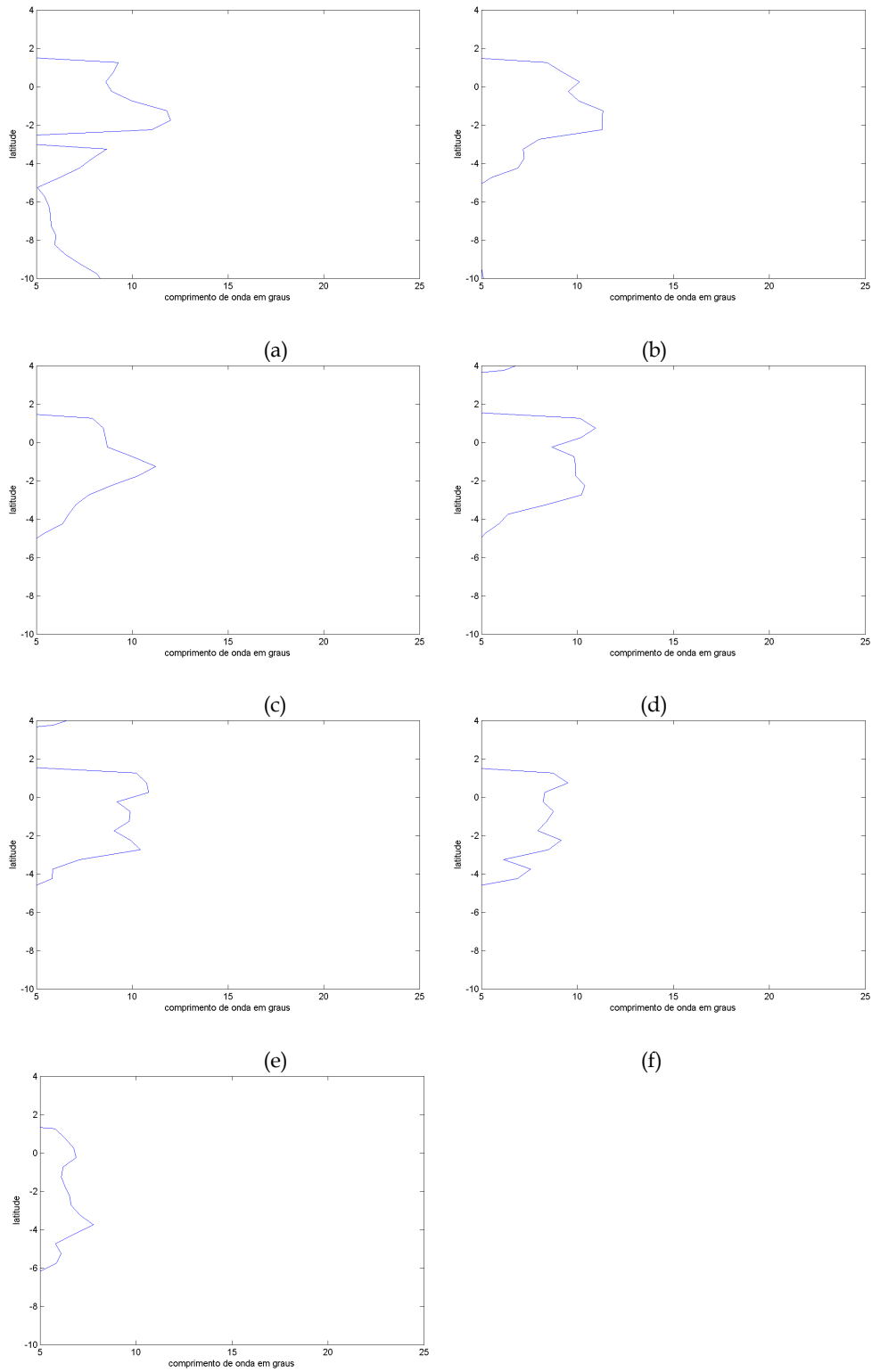
(g) Figura 4.49: Comprimento de onda dominante na região entre 15,25°W e 15,25°E, no sinal da componente zonal de corrente, filtrado entre 5 e 25° de longitude e 20 e 50 dias, a 15 (a), 35 (b), 46 (c), 83 (d), 96 (e), 148 (f) e 229 (g) metros de profundidade.
