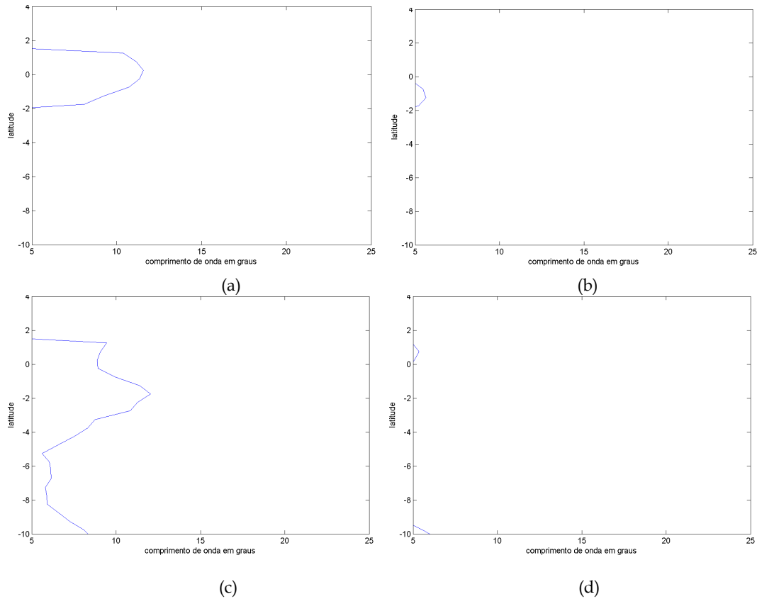
Figura 4.42: Comprimento de onda dominante (em graus), na região entre 15,25°W e 10,25°E, nos sinais de elevação da superfície livre (a), temperatura (b), componente zonal (c) e meridional (d) de corrente, filtrados entre 5 e 25° de longitude e 20 e 50 dias.
