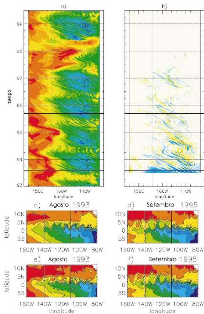
Figura 2.33: Diagrama de tempo x longitude de TSM ao longo de 2^{\circ} N, no experimento REF (a) e campo de diferença de TSM do experimento perturbado menos o REF (b). Campo de TSM para o experimento REF (c, d) e perturbado (e, f). Adaptado de: Vialard et al (2003).
