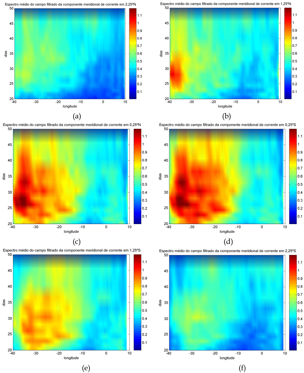
Figura 4.35: Espectro anual médio do campo da componente meridional de corrente, filtrado entre 5 e 25° de longitude e 20 e 50 dias, em 2,25°N (a), 1,25°N (b), 0,25°N (c), 0,25°S (d), 1,25°S (e) e 2,25°S (f).
