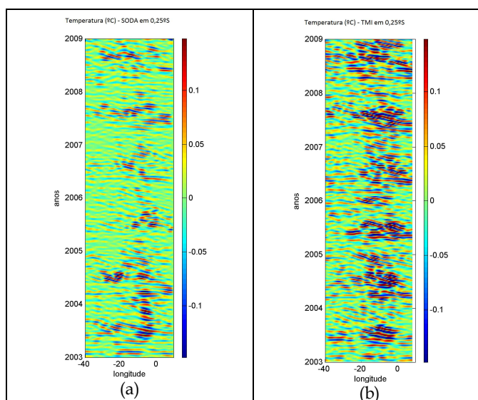
Figura 4.15: Temperatura na primeira camada (cerca de 5 metros de profundidade) do SODA (a) e TSM do TMI/AMSRE, ambos filtrados para o período entre 20 a 50 dias, e 5^{\circ} e 25^{\circ} de longitude, ao longo da latitude de 0,25^{\circ}\text{S} , entre 2003 e 2008.
