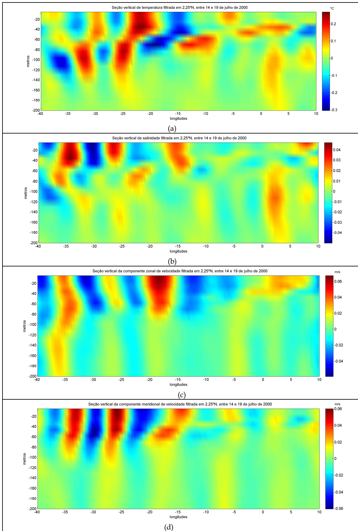
Figura 4.19: Seções verticais dos campos de temperatura (em graus Celsius) (a), salinidade (b), componente zonal (c) e meridional (d) (em m/s), filtrados para o período entre 20 a 50 dias, e 5° e 25° de longitude, ao longo da latitude de 2,25°N, entre os dias 14 e 19 de julho de 2000.
