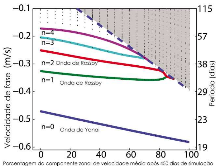
Figura 2.37: Relação entre a velocidade de fase e o período dos três modos livres obtidos da onda de 995km de comprimento, aumentando a intensidade do fluxo médio zonal de 0% a 100%. A linha pontilhada em azul representa a igualdade entre a velocidade de fase e a velocidade do fluxo médio. Adaptado de: Zhou e Boyd (2009).
