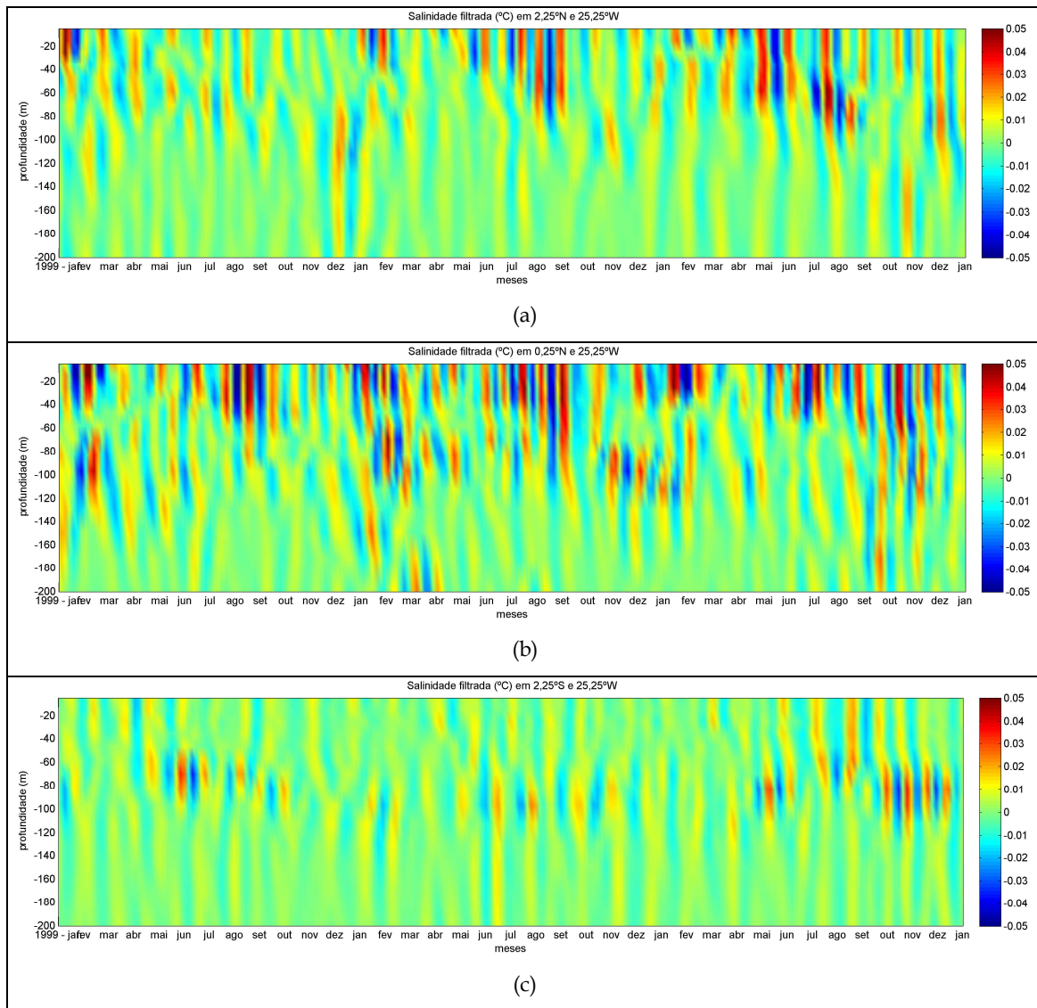
Figura 4.22: Perfis verticais ao longo do tempo dos campos filtrados de salinidade, sobre a longitude de 25,25°W e latitude de 2,25°N (a), 0,25°N (b) e 2,25°S (c), entre 1999 e 2002.
