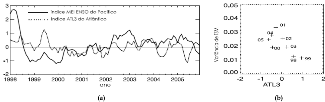
Figura 2.18: (a) Índices Multivariate ENSO Index (MEI) do Pacífico e ATL3 do Atlântico calculados para o período de 1998 a 2005 a partir da TSM do Tropical Rainfall Measuring Mission . (b) Variância das OITs no Atlântico, de junho a agosto na região entre 0^{\circ} a 35^{\circ}\text{W} e 0^{\circ} a 5^{\circ}\text{N} , em função do índice ATL3. Adaptado de: Wu e Bowman (2007a).
