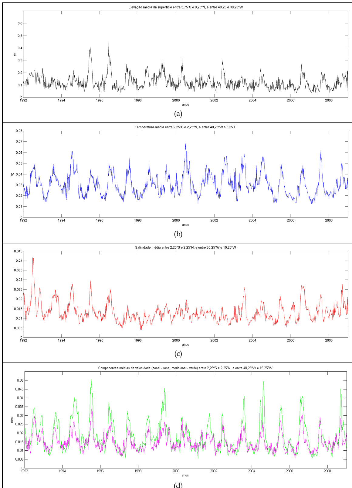
Figura 4.53: Valores médios das variáveis nas regiões de maior desvio padrão dos campos filtrados, entre os anos de 1992 e 2008. Média da elevação da superfície livre na região entre as os limites de 3,75°S a 0,25°N e 40,25°W a 30,25°W (a), média da temperatura entre os limites de 2,25°S a 2,25°N e 40,25°W a 8,25°E (b), média da salinidade entre os limites de 2,25°S a 2,25°N e 30,25°W a 10,25°W (c), e média das componentes zonal (rosa) e meridional (verde) da velocidade entre os limites de 2,25°S a 2,25°N e 40,25°W a 15,25°W.
