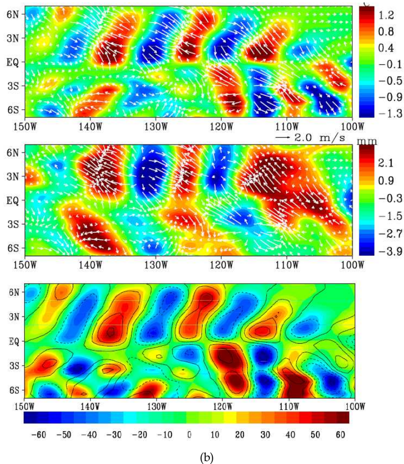
Figura 2.31: (a) Variações longitudinais em 3^{\circ}\text{N} em 11 de setembro de 1999, e a série temporal das anomalias filtradas de TSM, velocidade do vento em superfície, e as duas componentes da velocidade de corrente oceânica, em 3^{\circ}\text{N} , 135^{\circ}\text{W} . (b) Anomalias dos vetores de vento (setas brancas) sobrepostas às anomalias de TSM e vapor d'água (dois primeiros painéis), em 11 de setembro de 1999. O último painel em (b) é a anomalia de temperatura filtrada sobreposta (contorno, ^{\circ}\text{C} ) ao fluxo de calor latente (colorido, \text{W}/\text{m}^2 ) também em 11 de setembro de 1999. Adaptado de: Liu et al (2000).
