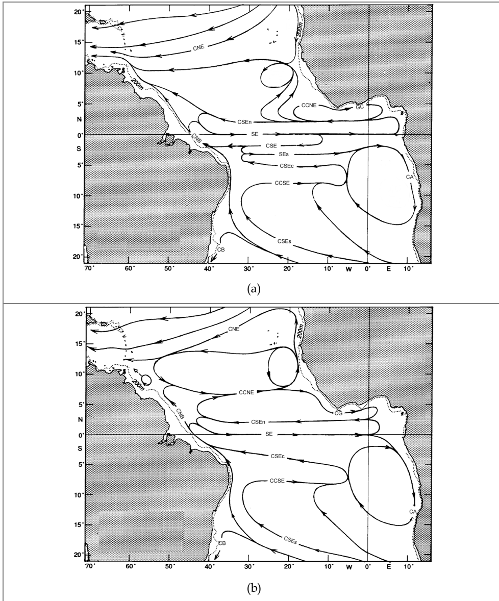
Figura 2.7: Mapa esquemático ilustrando a distribuição horizontal das principais correntes oceânicas superficiais (AT) do Atlântico, para outono (a) e primavera (b). Siglas: CNE – Corrente Norte Equatorial; CCNE – Contra-Corrente Norte Equatorial; CG – Corrente da Guiné; CSE – Corrente Sul Equatorial; CSEn – Corrente Sul Equatorial norte; CSEc – Corrente Sul Equatorial central; CSEs – Corrente Sul Equatorial sul; SE – Subcorrente Equatorial; CNB – Corrente Norte do Brasil; CA – Corrente da Angola; CCSE – Contra-Corrente Sul Equatorial; CB – Corrente do Brasil e SEs – Subcorrente Equatorial sul. Adaptado de: Stramma e Schott (1999).
