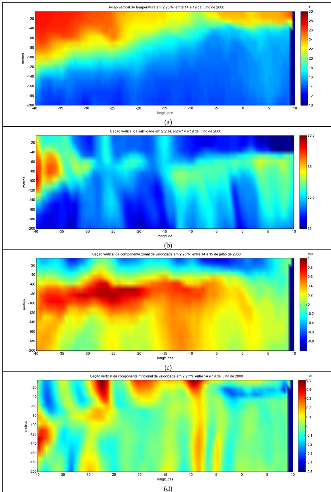
Figura 4.20: Seções verticais dos campos de temperatura (em graus Celsius) (a), salinidade (b), componente zonal (c) e meridional (d) (em m/s), ao longo da latitude de 2,25°N, entre os dias 14 e 19 de julho de 2000.
