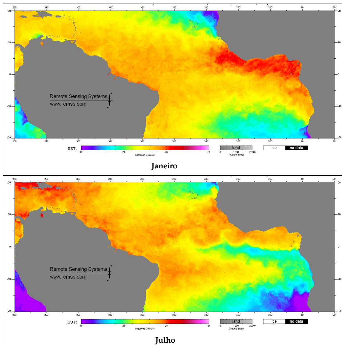
Figura 2.11: Campo de temperatura na superfície estimado pelo TMI ( Tropical Rainfall Measuring Mission Microwave Imager ), exemplificando a presença da pluma de água fria durante o mês de Julho e ausente em Janeiro (2009). Disponível em: www.remss.com/sst/sst_data_daily.html
