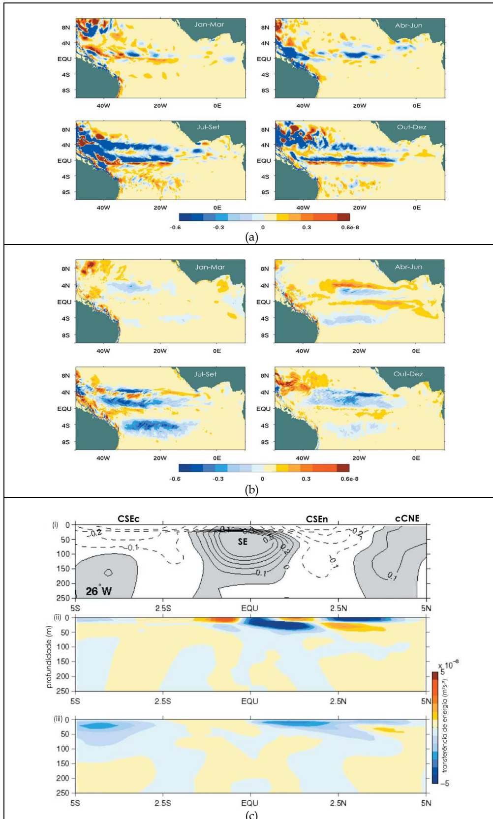
Figura 2.19: Mapas sazonais da taxa de produção de instabilidade barotrópica (a) e baroclínica (b) ( m^2s^{-3} ), média dos 6 anos de simulação e dos primeiros 50 metros de profundidade. Valores negativos significam transferência de energia do fluxo médio para a perturbação (a) e da energia potencial de perturbação para a energia cinética de perturbação (b). (c) Estrutura vertical das correntes médias zonais (i), Taxa de produção barotrópica (ii) e baroclínica (iii) média entre 30°W a 10°W. Adaptado de: von Schuckman et al (2008).
