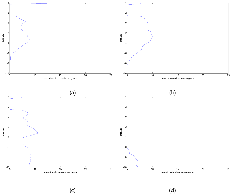
Figura 4.48: Comprimento de onda dominante (em graus) na região entre 15,25°W e 15,25°E, no sinal de salinidade, filtrado entre 5 e 25° de longitude e 20 e 50 dias, a 83 (a), 96 (b), 148 (c) e 229 (d) metros de profundidade.
