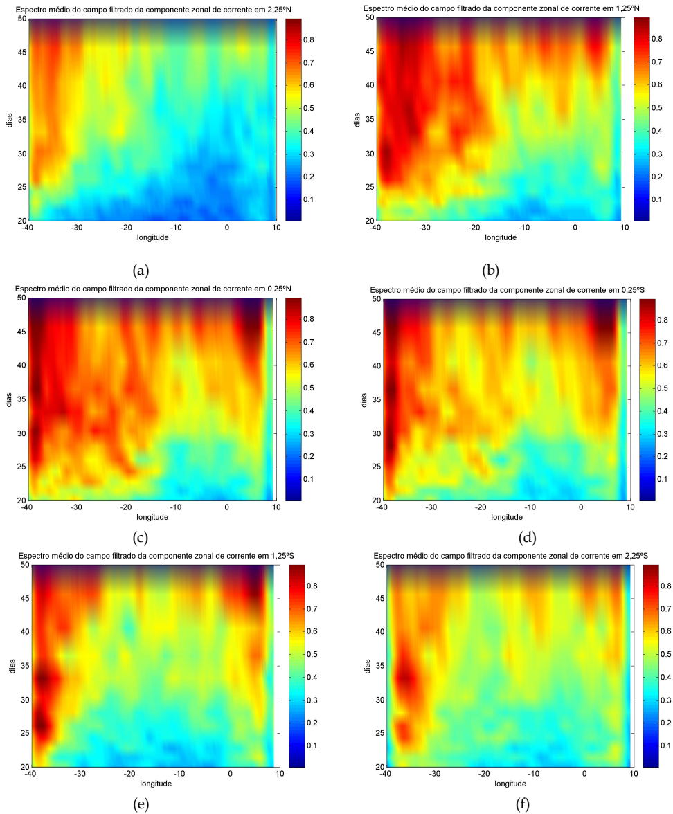
Figura 4.34: Espectro anual médio do campo da componente zonal de corrente, filtrado entre 5 e 25^{\circ} de longitude e 20 e 50 dias, em 2,25^{\circ}\text{N} (a), 1,25^{\circ}\text{N} (b), 0,25^{\circ}\text{N} (c), 0,25^{\circ}\text{S} (d) 1,25^{\circ}\text{S} (e) e 2,25^{\circ}\text{S} (f).
