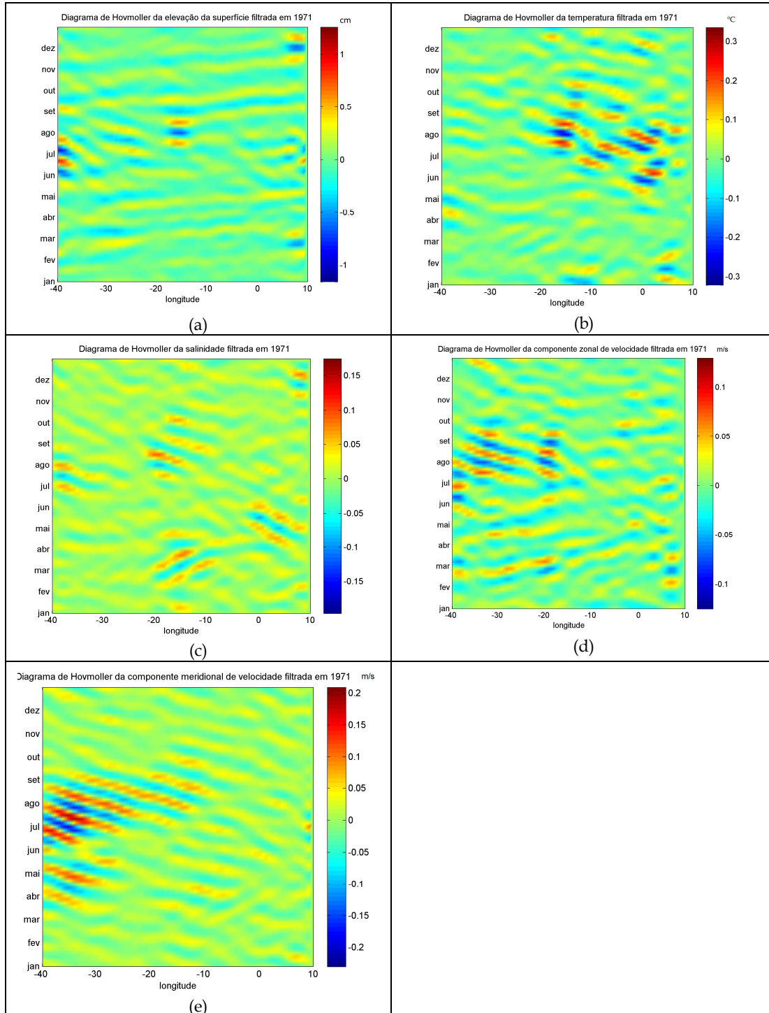
Figura 4.9: Diagramas de Hovmöller dos resultados do SODA, filtrados para o período entre 20 a 50 dias, e 5^{\circ} e 25^{\circ} de longitude, na primeira camada (cerca de 5 metros de profundidade), ao longo da latitude de 0,25^{\circ}\text{N} , durante o ano de 1971. (a) elevação da superfície livre (cm), (b) temperatura ( ^{\circ}\text{C} ), (c) salinidade (d) componente zonal (m/s) e (e) meridional da velocidade (m/s).
