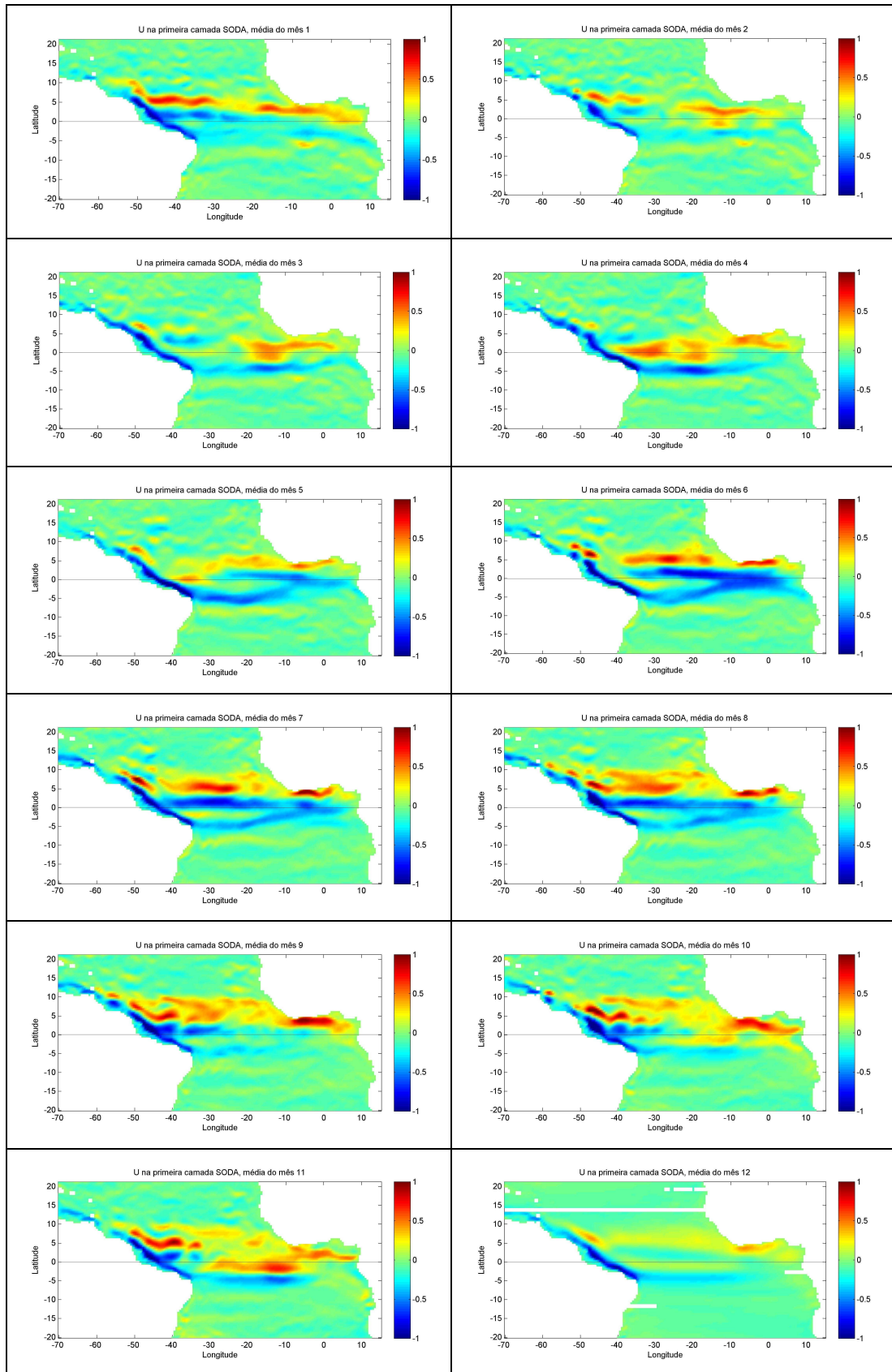
Figura 4.6: Médias mensais da componente zonal de velocidade na primeira camada do SODA.
