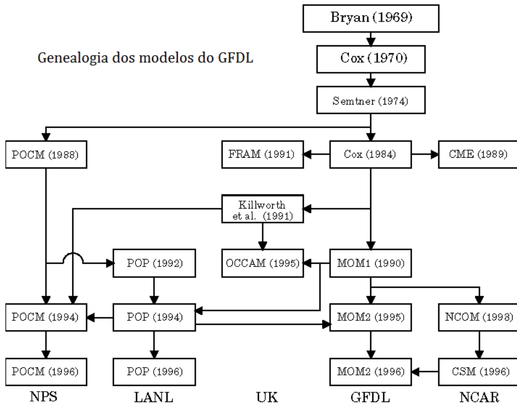
Figura 3.1: Organograma do histórico dos modelos do GFDL ( Geophysical Fluid Dynamics Laboratory ) e a origem do POP ( Parallel Ocean Program ). Fonte: http://climate.lanl.gov/Models/POP/
