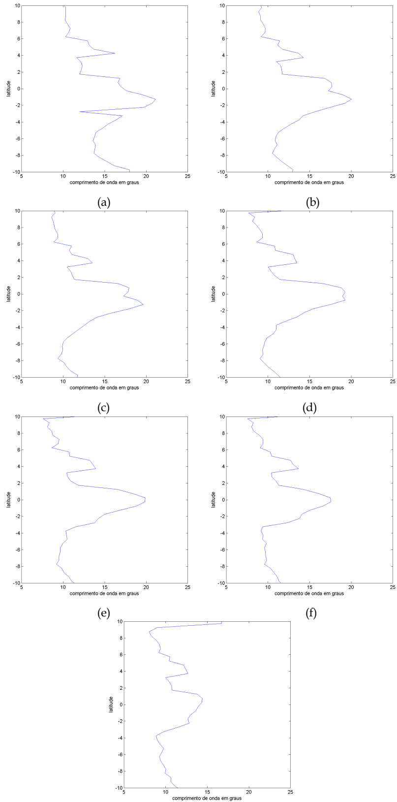
(g) Figura 4.45: Comprimento de onda dominante (em graus) na região entre 40,25^{\circ}\text{W} e 10,25^{\circ}\text{W} , no sinal da componente zonal de corrente, filtrado entre 5 e 25^{\circ} de longitude e 20 e 50 dias, a 15 (a), 35 (b), 46 (c), 83 (d), 96 (e), 148 (f) e 229 (g) metros de profundidade.
