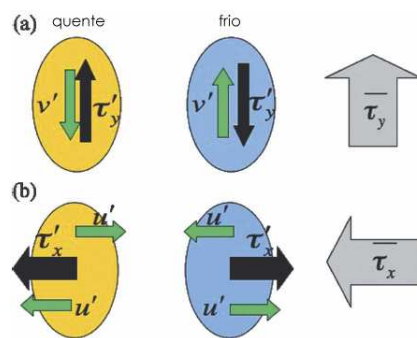
Figura 2.17: Representação esquemática da interação do atrito de vento, correntes superficiais e TSM. A cor azul (amarelo) representa água fria (quente). As setas cinza são os campos de vento; as pretas, a perturbação do vento gerada pelas TIWs; e as verdes são as perturbações de correntes superficiais. Fonte: Seo et al (2007).
