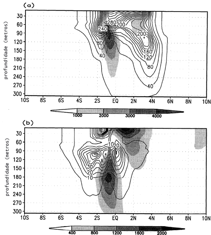
Figura 2.27: Seções verticais da média temporal de energia cinética (sombreado) e média temporal da energia cinética turbulenta (contorno), em 130°W (a) e em 170°W (b). Adaptado de: Masina et al (1999).
