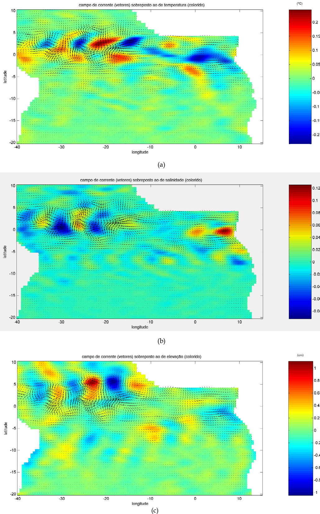
Figura 4.18: Campos dos resultados do SODA filtrados para o período entre 20 a 50 dias, e 5° e 25° de longitude, na primeira camada (cerca de 5 metros de profundidade), entre os dias 14 e 19 de julho de 2000. (a) Em cores está a temperatura (°C), os contornos pretos representam a elevação da superfície livre (intervalo de 0,002 m) e as setas correspondem às correntes. (b) O mesmo que em (a), exceto que o campo colorido representa a salinidade. (c) Comparação entre o campo de temperatura (cores, °C) e salinidade (contorno preto).
