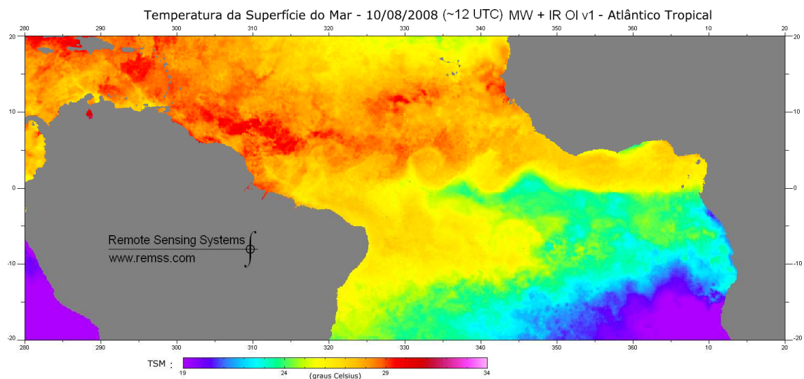
Figura 1.1: Campo de temperatura na superfície do mar, estimado pelo TMI ( Tropical Rainfall Measuring Mission Microwave Imager ), para o dia 10 de agosto de 2008. Disponível em: www.remss.com/sst/sst_data_daily.html
