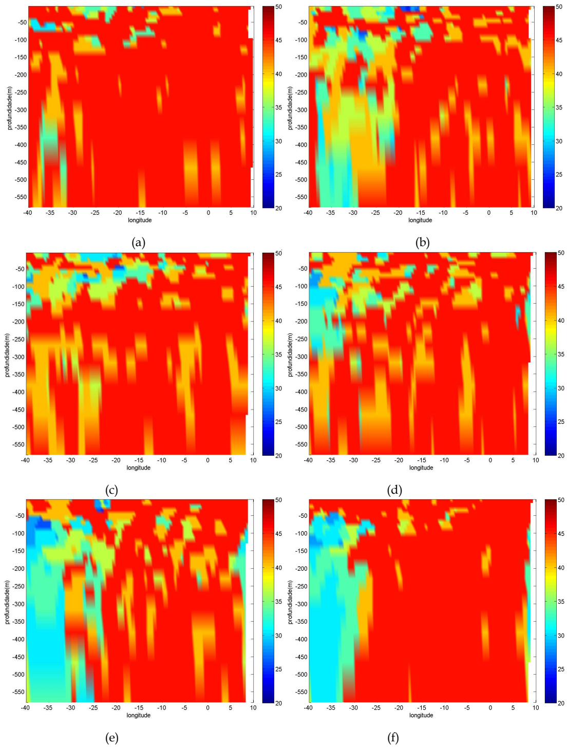
Figura 4.36: Períodos dominantes (em dias) no sinal de temperatura filtrado entre 5 e 25° de longitude e 20 e 50 dias, nas seções verticais ao longo da latitude de 2,2,5°N (a), 1,25°N (b), 0,25°N (c), 0,25°S (d), 1,25°S (e) e 2,25°S (f).
