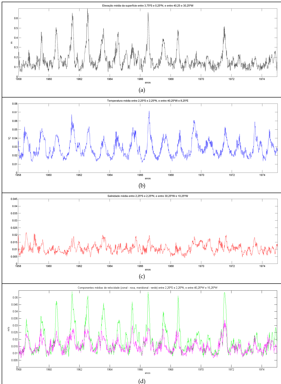
Figura 4.51: Valores médios das variáveis nas regiões de maior desvio padrão dos campos filtrados, entre os anos de 1958 e 1974. Média da elevação da superfície livre na região entre as os limites de 3,75°S a 0,25°N e 40,25°W a 30,25°W (a), média da temperatura entre os limites de 2,25°S a 2,25°N e 40,25°W a 8,25°E (b), média da salinidade entre os limites de 2,25°S a 2,25°N e 30,25°W a 10,25°W (c), e média das componentes zonal (rosa) e meridional (verde) da velocidade entre os limites de 2,25°S a 2,25°N e 40,25°W a 15,25°W.
