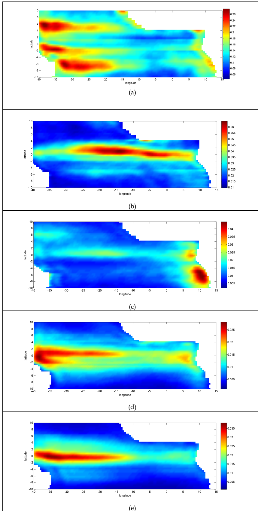
Figura 4.25: Desvio padrão do sinal das OITs nos resultados do SODA filtrados para o período entre 20 a 50 dias, e 5^{\circ} e 25^{\circ} de longitude, na primeira camada (cerca de 5 metros de profundidade). (a) elevação da superfície livre (m), (b) temperatura ( ^{\circ}\text{C} ), (c) salinidade (d) componente zonal (m/s) e (e) meridional da velocidade (m/s). Variação para os 51 anos de simulação.
