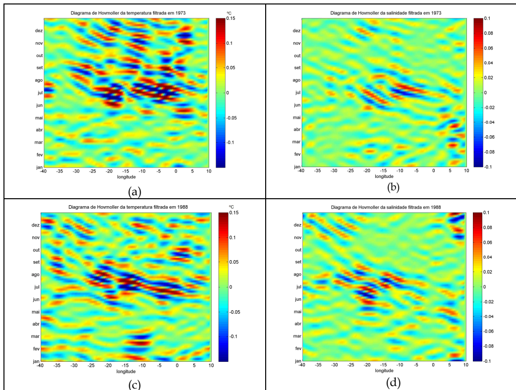
Figura 4.12: Diagramas de Hovmöller dos resultados do SODA, filtrados para o período entre 20 a 50 dias, e 5^{\circ} e 25^{\circ} de longitude, na primeira camada (cerca de 5 metros de profundidade), ao longo da latitude de 0,25^{\circ}\text{N} , durante os anos de 1973 na (a) temperatura ( ^{\circ}\text{C} ) e (b) salinidade, e de 1988 na (a) temperatura ( ^{\circ}\text{C} ) e (b) salinidade.
