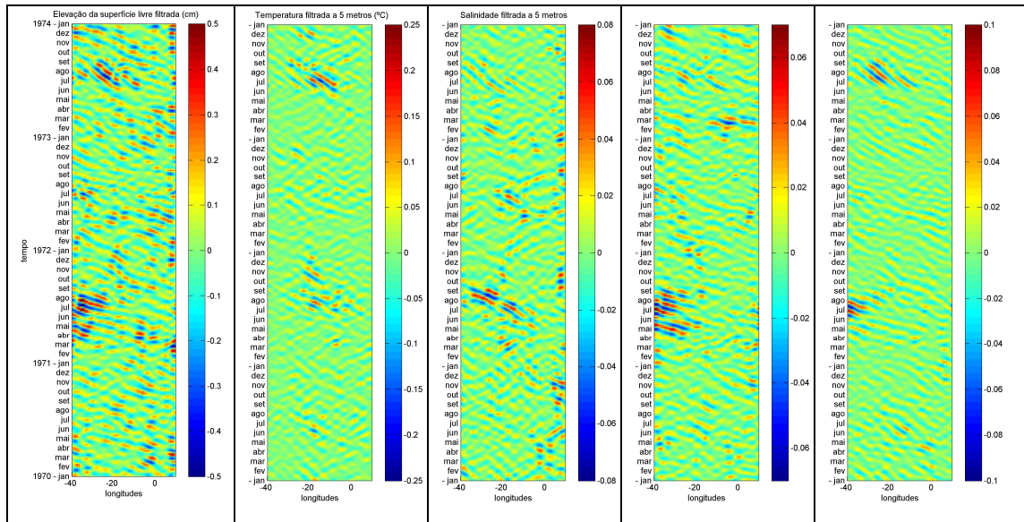
Figura 4.13: Diagramas de Hovmöller dos resultados do SODA, filtrados para o período entre 20 a 50 dias, e 5^{\circ} e 25^{\circ} de longitude, na primeira camada (cerca de 5 metros de profundidade), na latitude de 2,25^{\circ}\text{N} , ao longo do tempo (entre 1968 e 1972). (a) elevação da superfície livre (cm), (b) temperatura ( ^{\circ}\text{C} ), (c) salinidade (d) componente zonal (m/s) e (e) meridional da velocidade (m/s).
