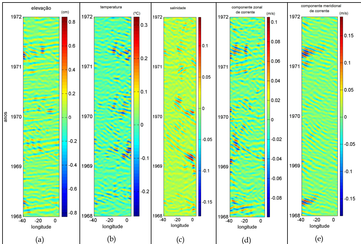
Figura 4.8: Diagramas de Hovmöller dos resultados do SODA, filtrados para o período entre 20 a 50 dias, e 5^{\circ} e 25^{\circ} de longitude, na primeira camada (cerca de 5 metros de profundidade), na latitude de 0,25^{\circ}\text{N} , ao longo do tempo (entre 1968 e 1972). (a) elevação da superfície livre (cm), (b) temperatura ( ^{\circ}\text{C} ), (c) salinidade (d) componente zonal (m/s) e (e) meridional da velocidade (m/s).
