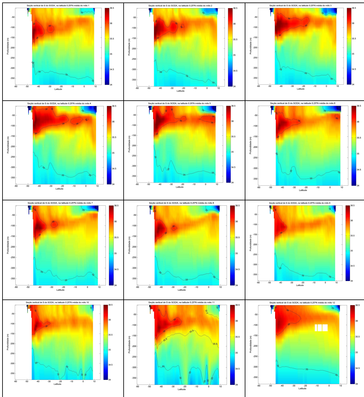
Figura 4.4. Médias mensais de salinidade gerada pelo SODA na seção zonal vertical ao longo da latitude de 0,25^{\circ}\text{N} .
