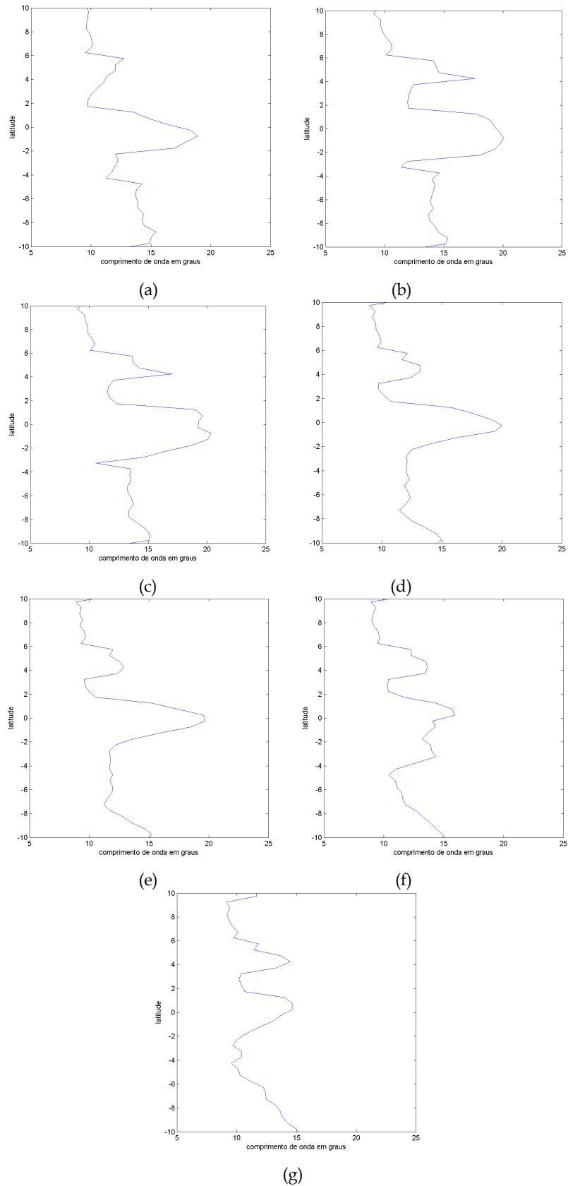
Figura 4.43: Comprimento de onda dominante (em graus) na região entre 40,25^{\circ}\text{W} e 10,25^{\circ}\text{W} , no sinal de temperatura, filtrado entre 5 e 25^{\circ} de longitude e 20 e 50 dias, a 15 (a), 35 (b), 46 (c), 83 (d), 96 (e), 148 (f) e 229 (g) metros de profundidade.
