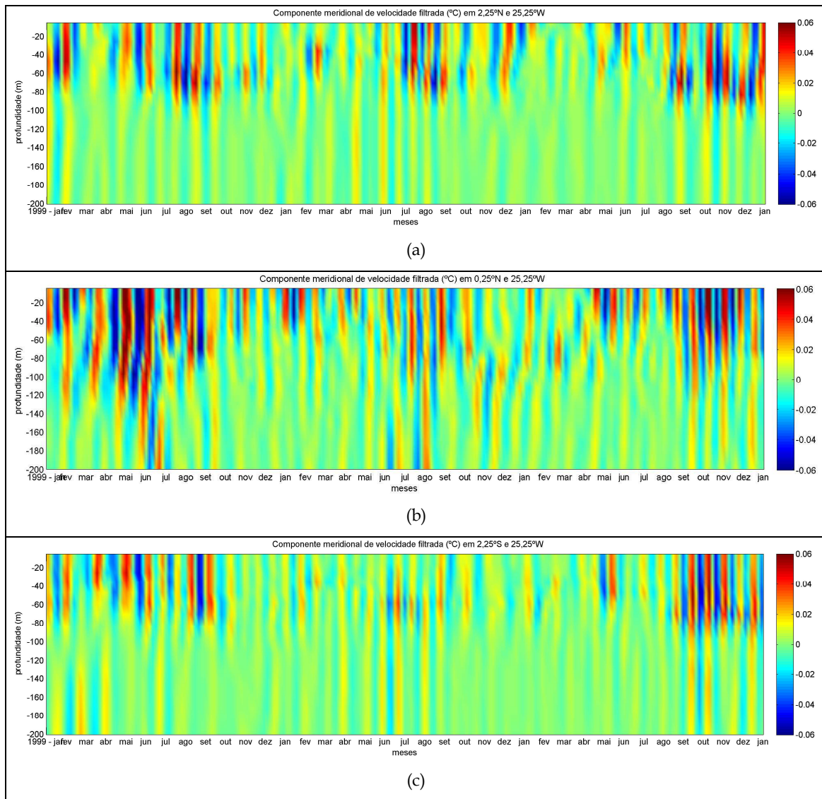
Figura 4.24: Perfis verticais ao longo do tempo dos campos filtrados da componente meridional de velocidade (m/s), sobre a longitude de 25,25°W e latitude de 2,25°N (a), 0,25°N (b) e 2,25°S (c), entre 1999 e 2002.
