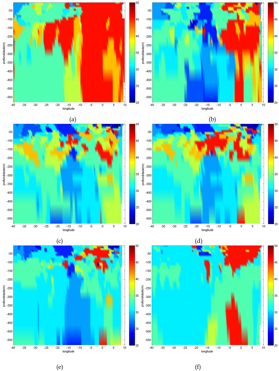
Figura 4.39: Período dominante (em dias) no sinal da componente zonal de corrente, filtrado entre 5 e 25° de longitude e 20 e 50 dias, nas seções verticais ao longo da latitude de 2,25^{\circ}\text{N} (a), 1,25^{\circ}\text{N} (b), 0,25^{\circ}\text{N} (c), 0,25^{\circ}\text{S} (d), 1,25^{\circ}\text{S} (e) e 2,25^{\circ}\text{S} (f).
