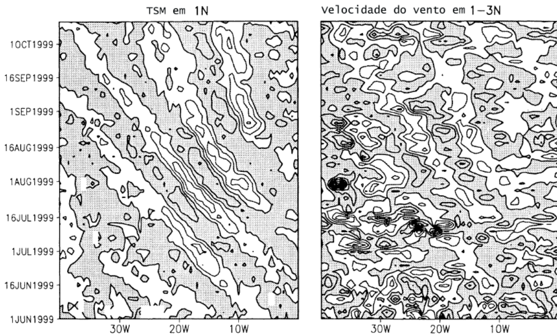
Figura 2.13: Seções de longitude x tempo de anomalia de TSM em 1°N e velocidade do vento. Adaptado de: Hashizume et al (2001).
