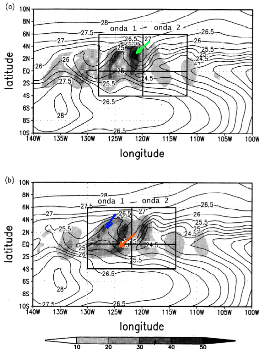
Figura 2.29: Gráfico no tempo t = 3 dias (a) e 9 dias (b) da distribuição de energia cinética turbulenta (sombreado) e TSM (contorno). Adaptado de: Masina et al (1999).
