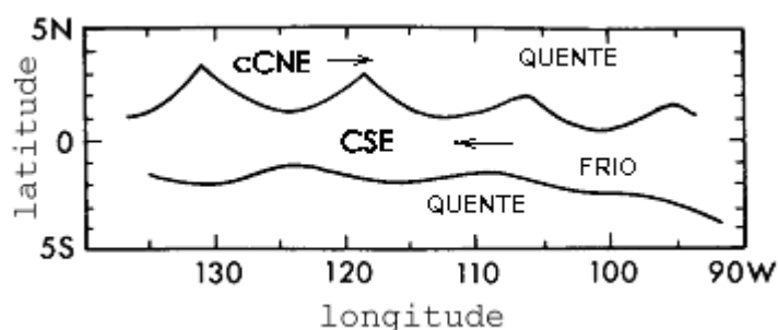
Figura 2.12: Representação esquemática do padrão de TSM e correntes oceânicas da região equatorial. Adaptado de: Philander (1976).
