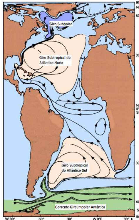
Figura 2.6: Principais giros de circulação oceânica superficial do Atlântico. Adaptado de: Tomczak e Godfrey (2005).
