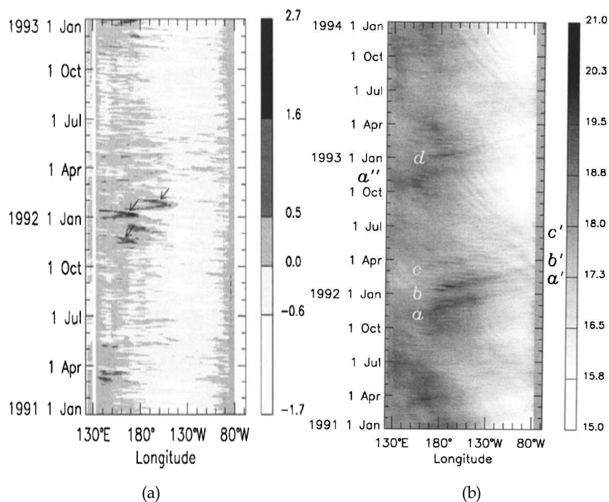
Figura 2.21: Gráfico tempo x longitude da componente zonal dos ventos (a) e da temperatura (b) ao longo de 2°N extraída da simulação a , b e c denotam as ondas de Kelvin, geradas pelas rajadas de vento de oeste, que excitam ondas de Rossby ( a' , b' e c' ) ao refletir na fronteira leste. Fonte: Lawrence et al (1998).
