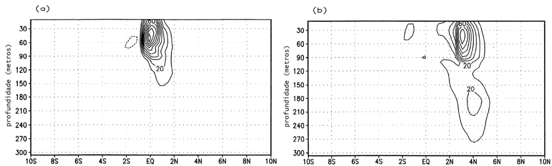
Figura 2.28: Seções verticais em 130°W da média temporal de conversão barotrópica (a) e conversão baroclínica (b). Adaptado de: Masina et al (1999).
