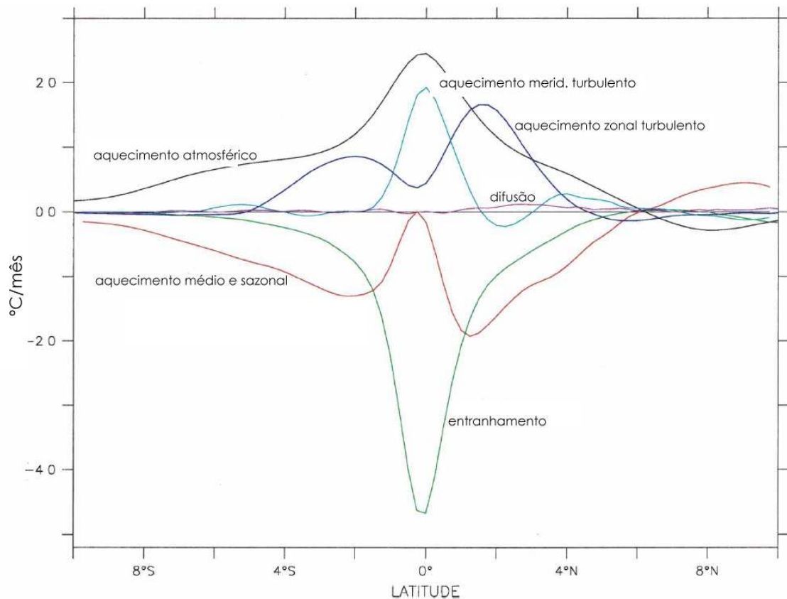
Figura 2.36: Balanço médio anual de temperatura para o Pacífico tropical entre 145 e 135°W. Preto: fluxo de calor na superfície, vermelho: advecção média e sazonal de temperatura, azul escuro: advecção turbulenta zonal de temperatura, azul claro: advecção turbulenta meridional de temperatura, verde: entranhamento, lilás: difusão. Adaptado de: Jochum e Murtugudde (2006).
