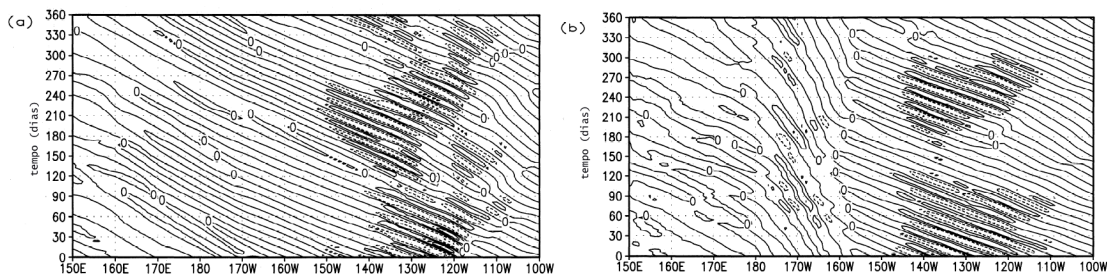
Figura 2.24: Diagrama de Hovmöller de velocidade meridional perturbada (velocidade total menos a média do ano inteiro) a 95 metros de profundidade em 2°N (a) e 2°S (b). Adaptado de: Masina e Philander (1999).
